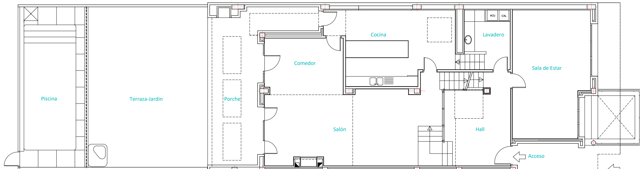
Planta de Acceso y Salones
