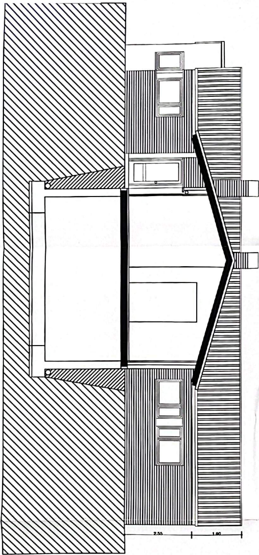
SECCIO C-C'
