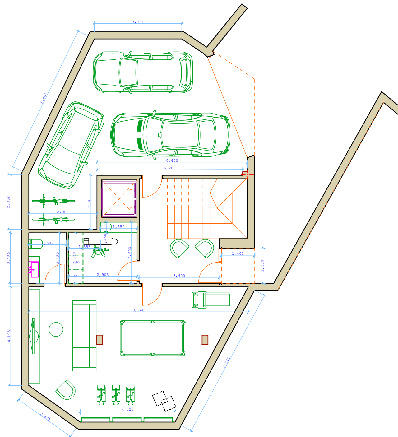
0. Planta Soterrani Cotes 1:100
