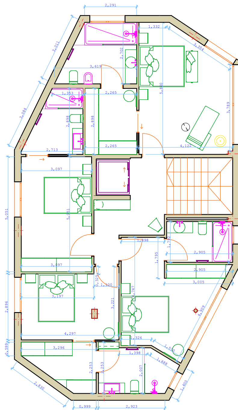
0. Planta Baixa Habitatge Cotes 1:100
