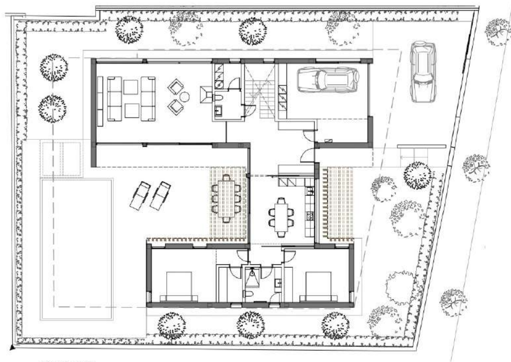
PLANTA BAIXA
