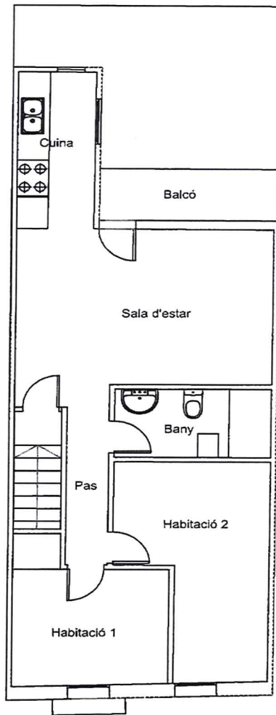
PLANTA PIS
