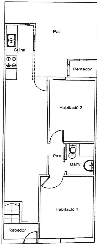
PLANTA BAIXA
