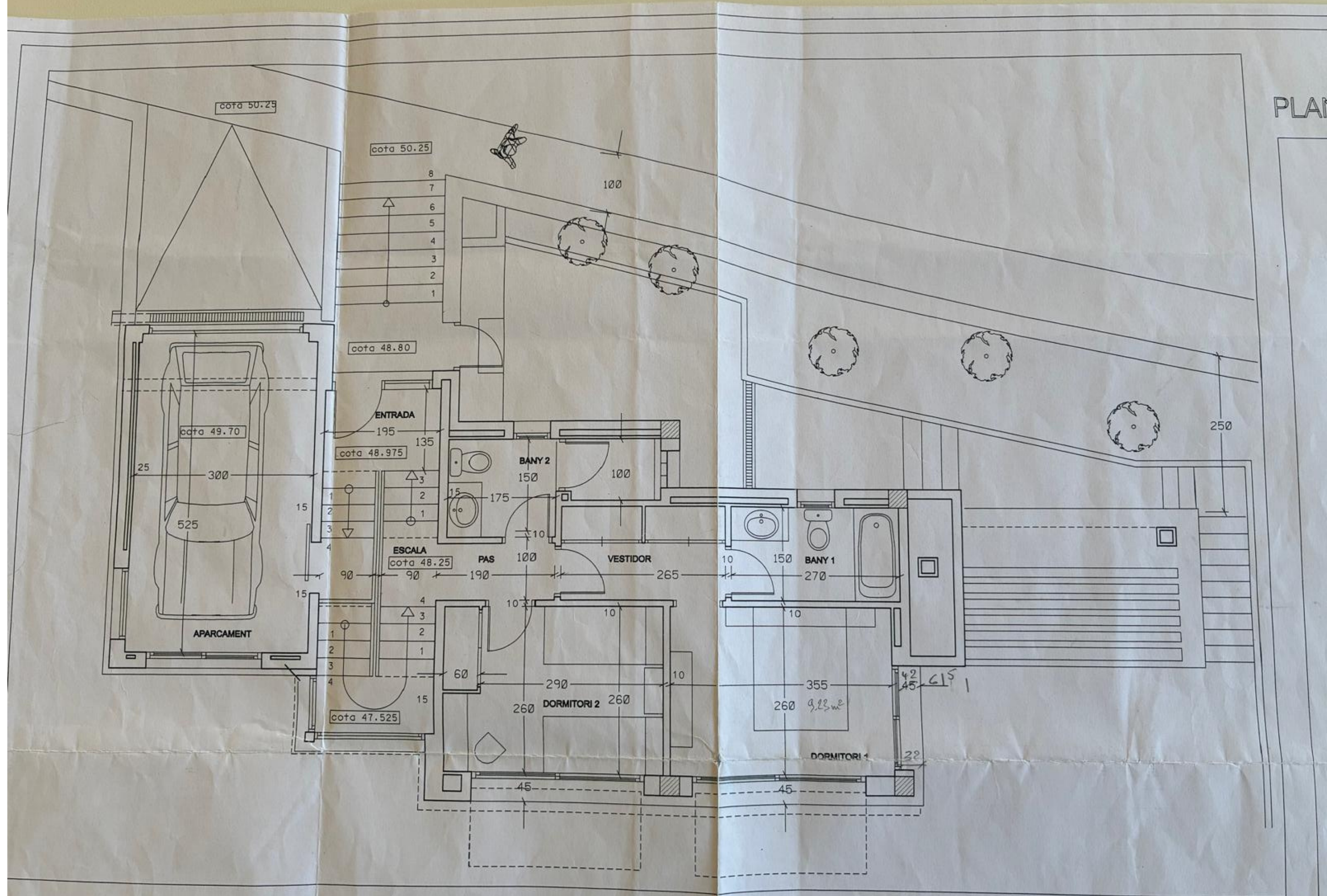
PLANTA PRIMERA
