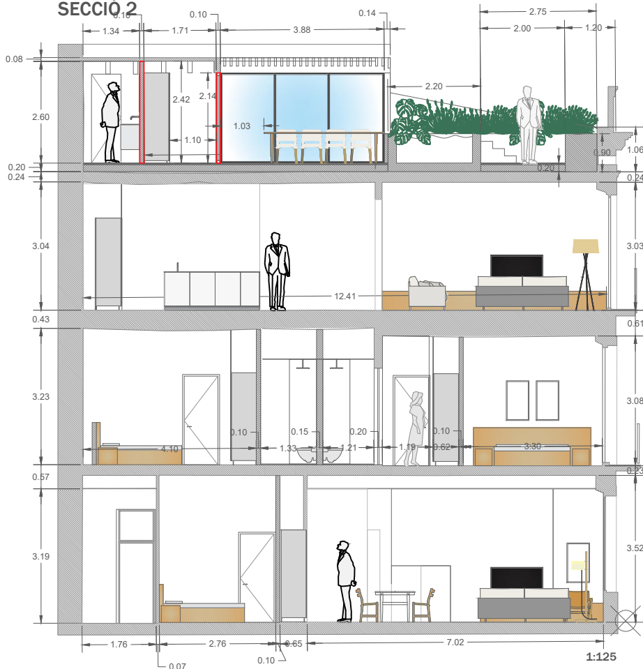
SECCIÓ 2
