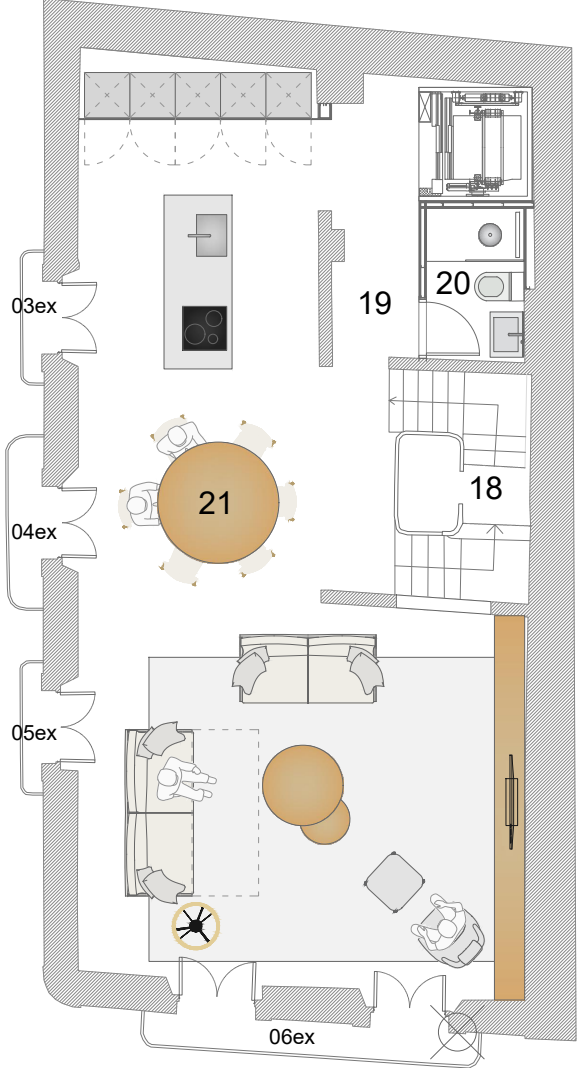
PLANTA SEGONA
