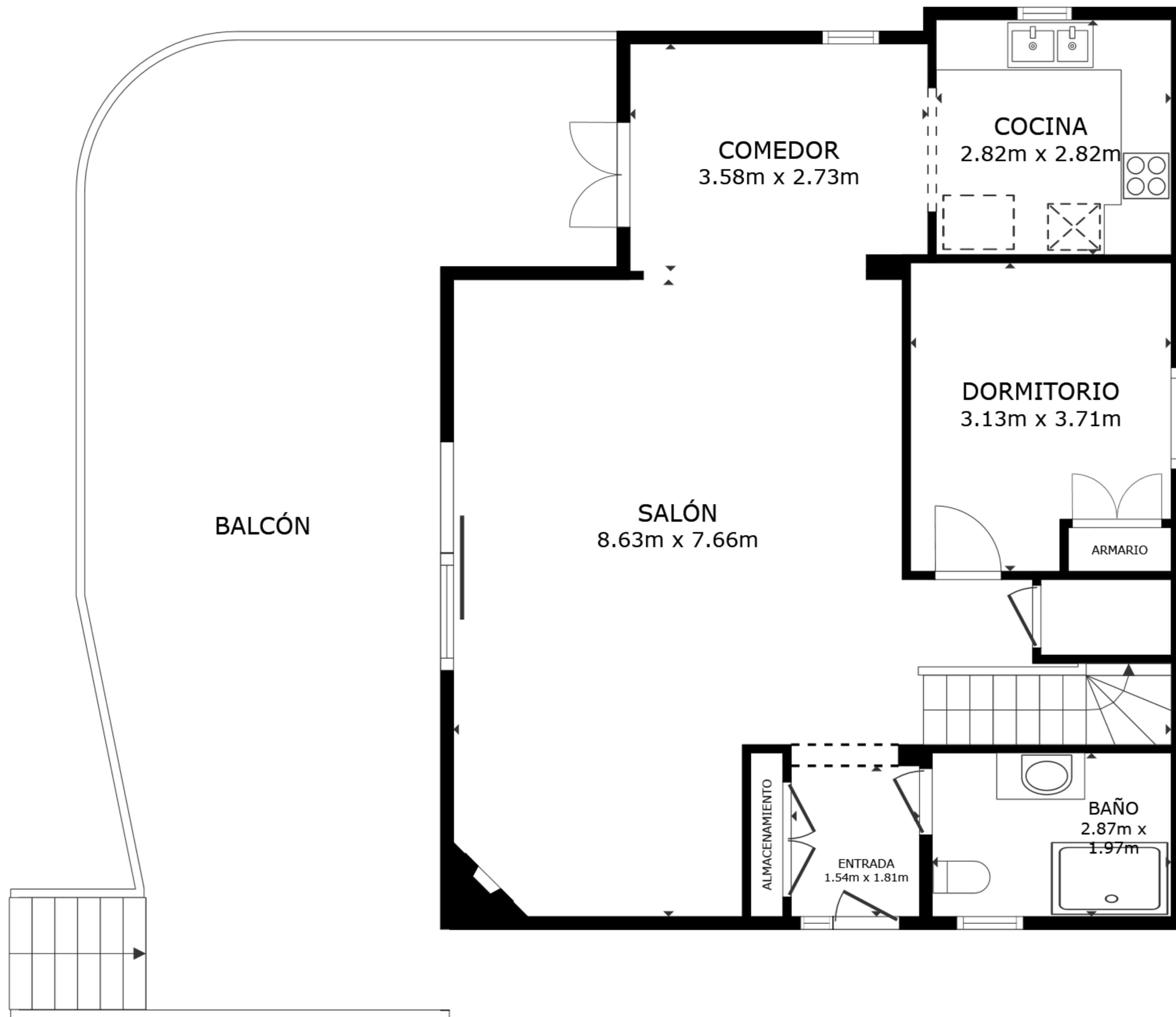
PLANTA 1
