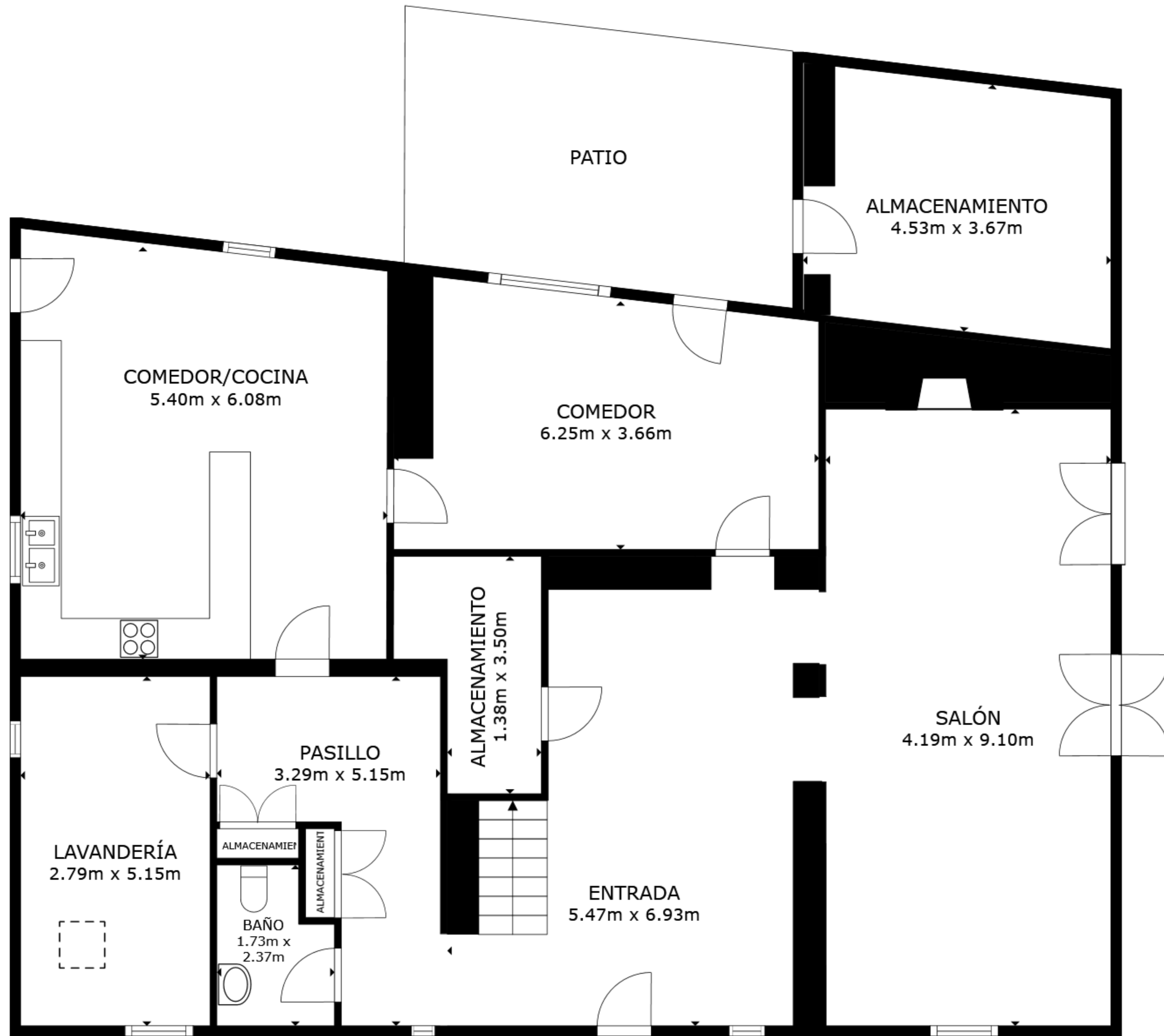
PLANTA 1
