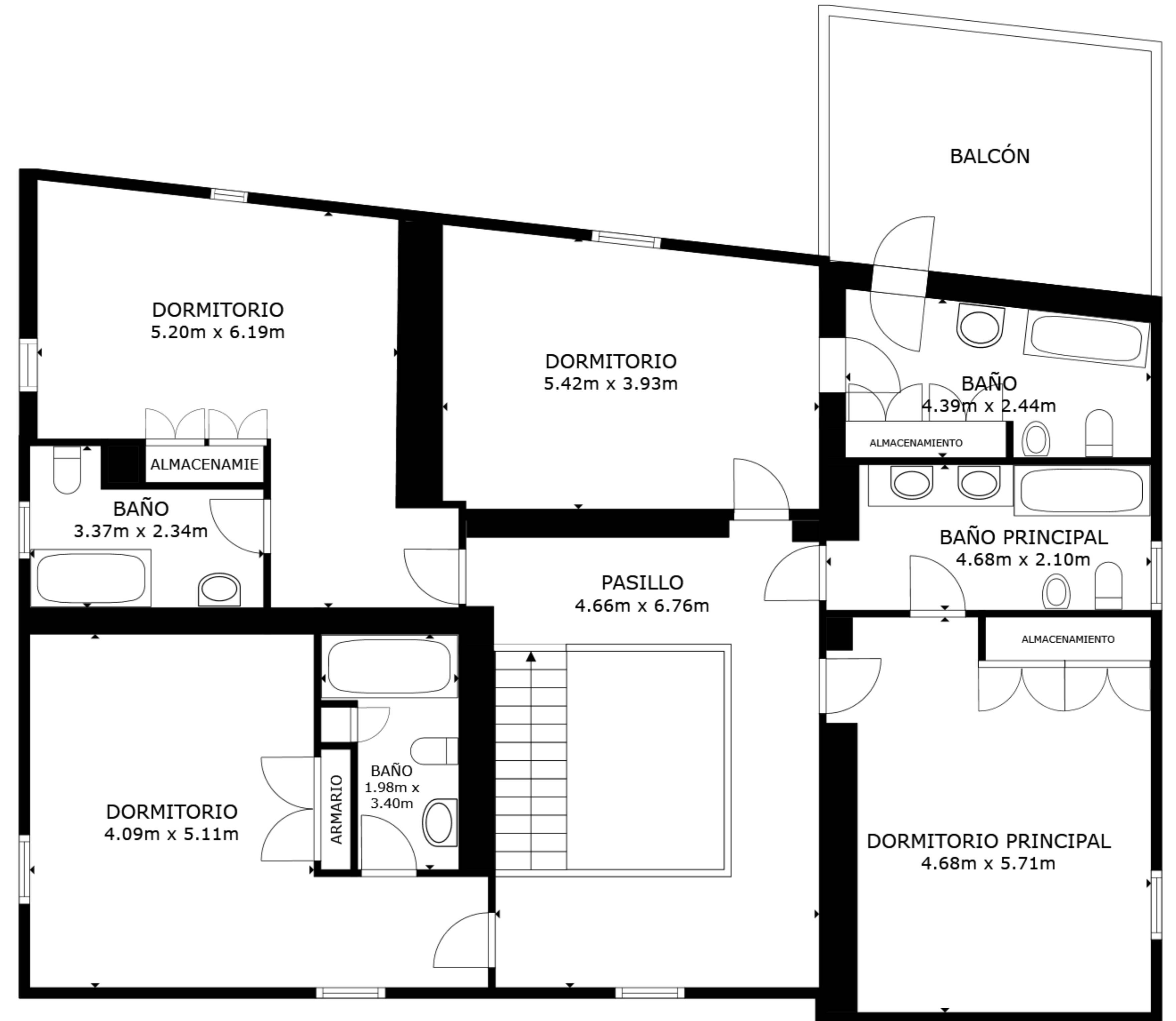
PLANTA 2
