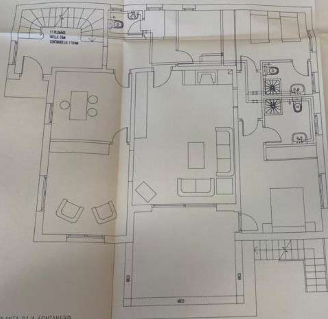
PLANTA BAJA FONTANERIA
