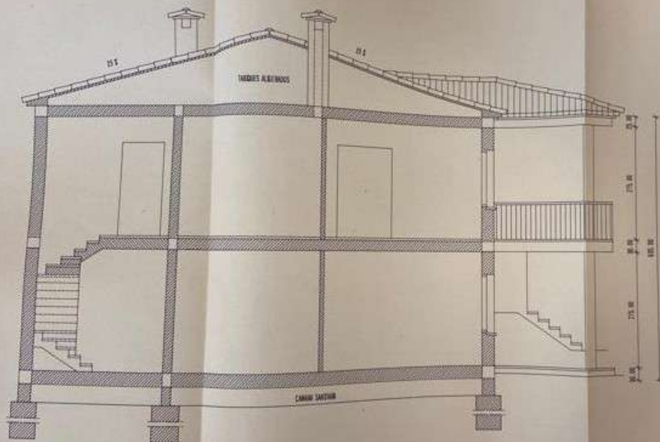
SECCION A-A'
