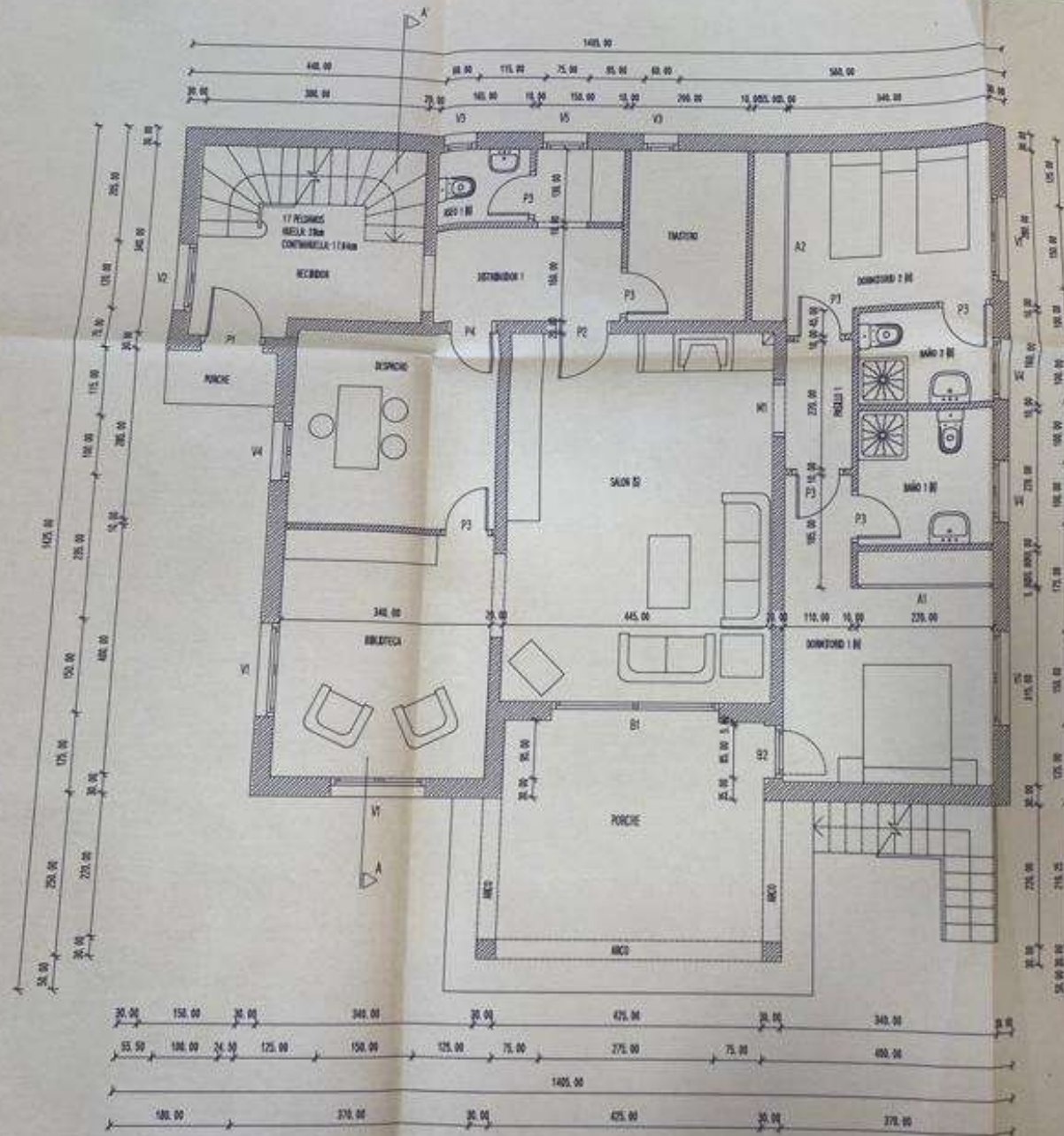
PLANTA BAJA
