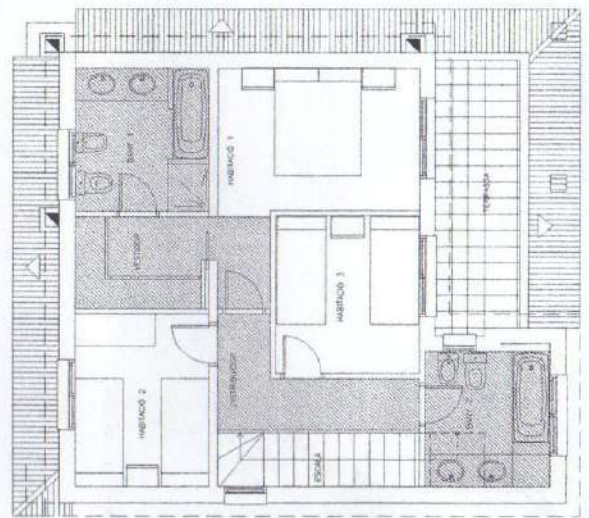
PLANTA PIS_2
