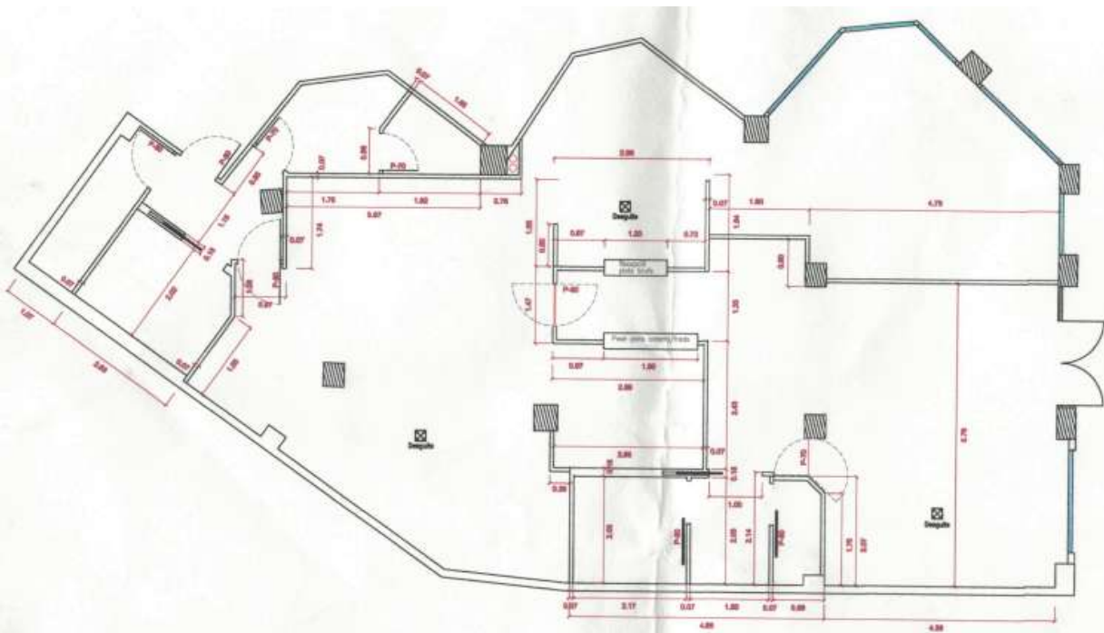
DETALLI PLANTA
