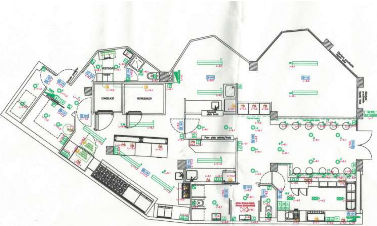
PLANOL ELÈCTRIC
