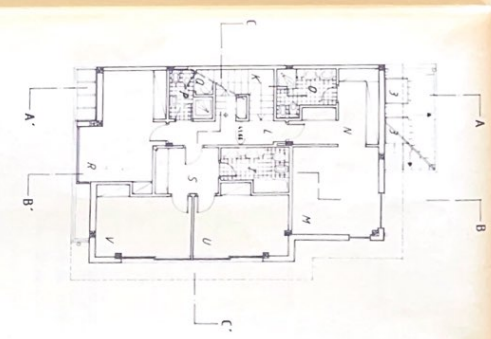
1º ANDAR
