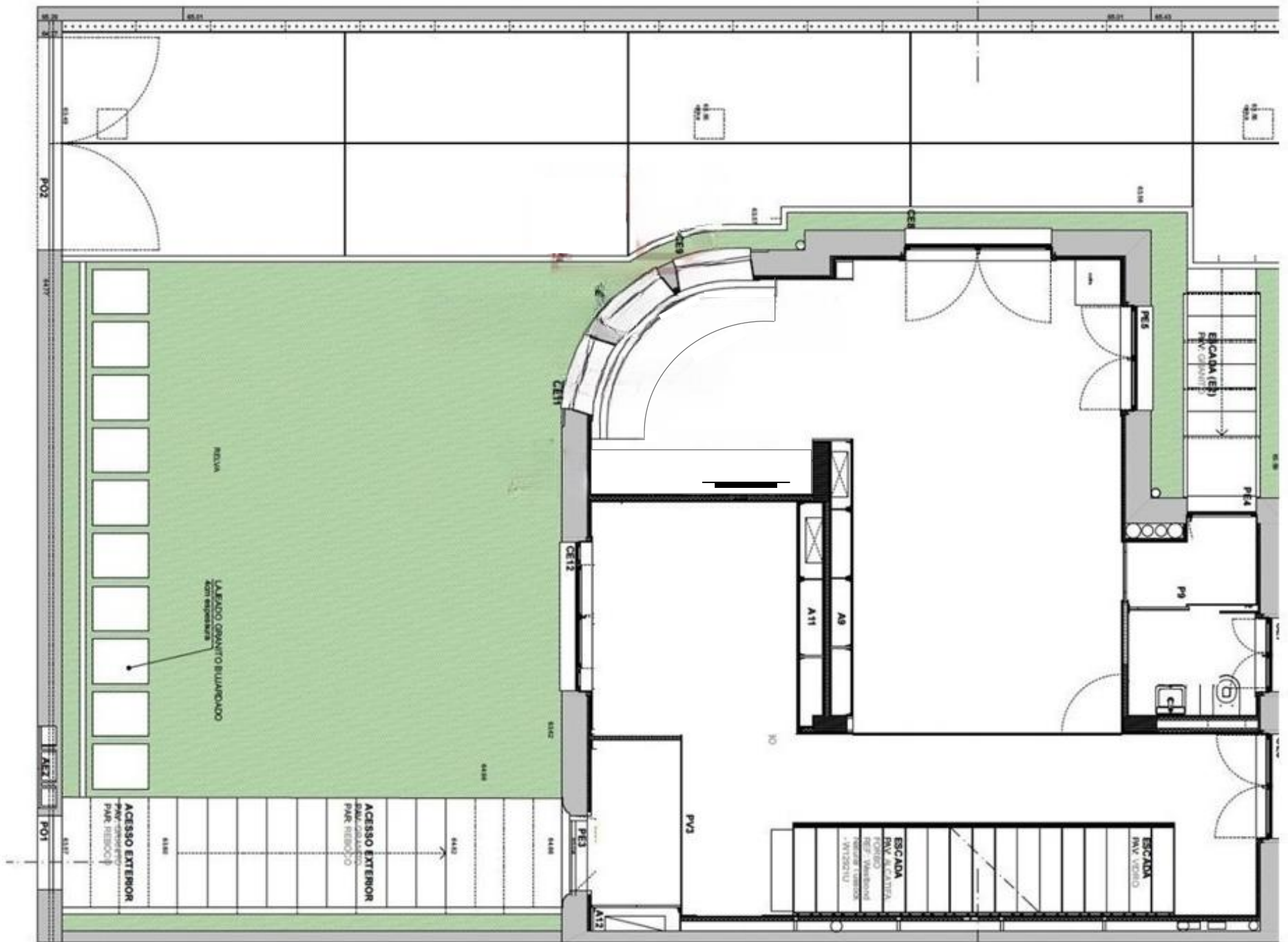
PLANTA PISO 0 - ESCALA 1:50
