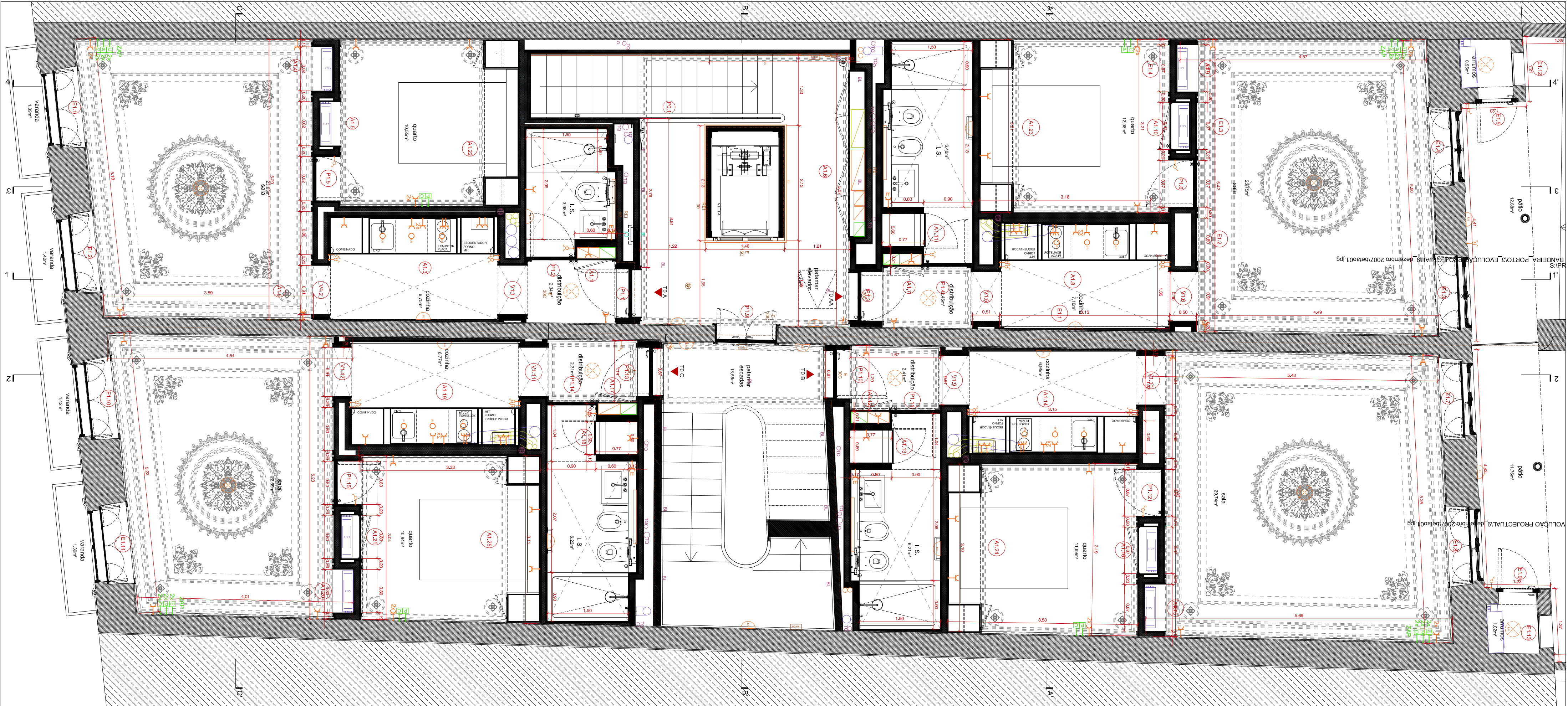
PLANTA 1º ANDAR
