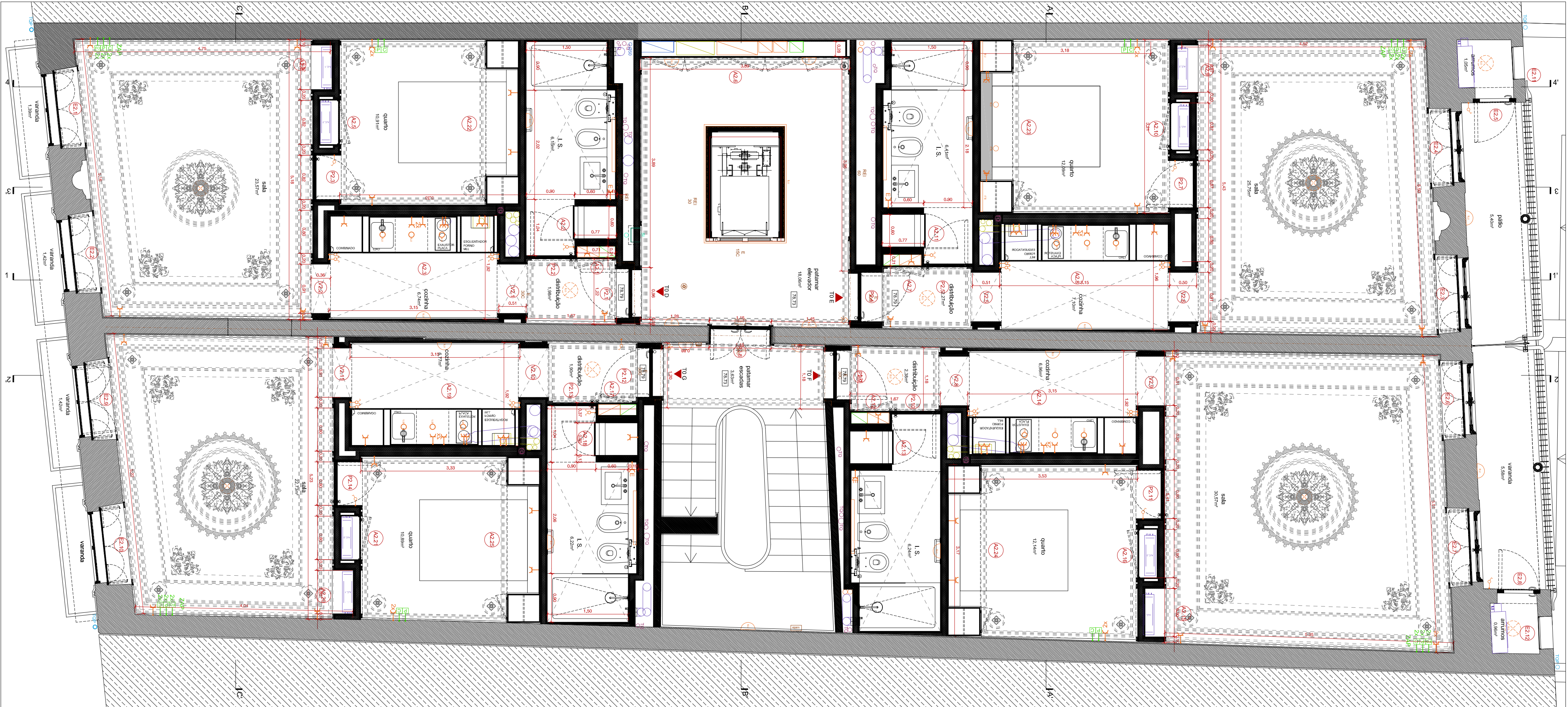
PLANTA 2º ANDAR
