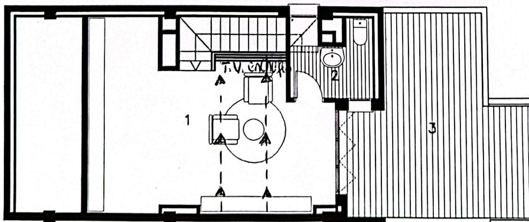
Planta Sotacoberta
