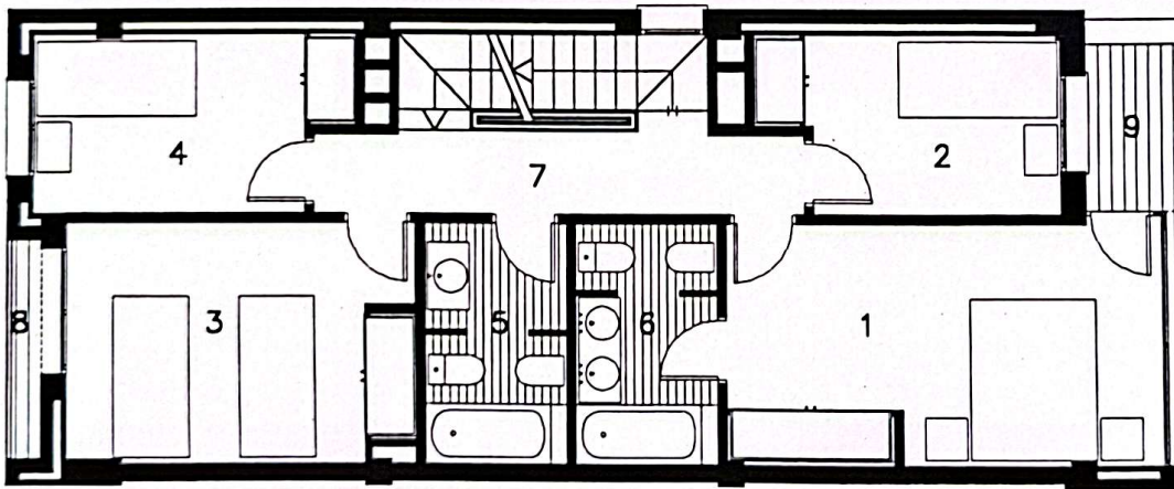
Planta Primera
