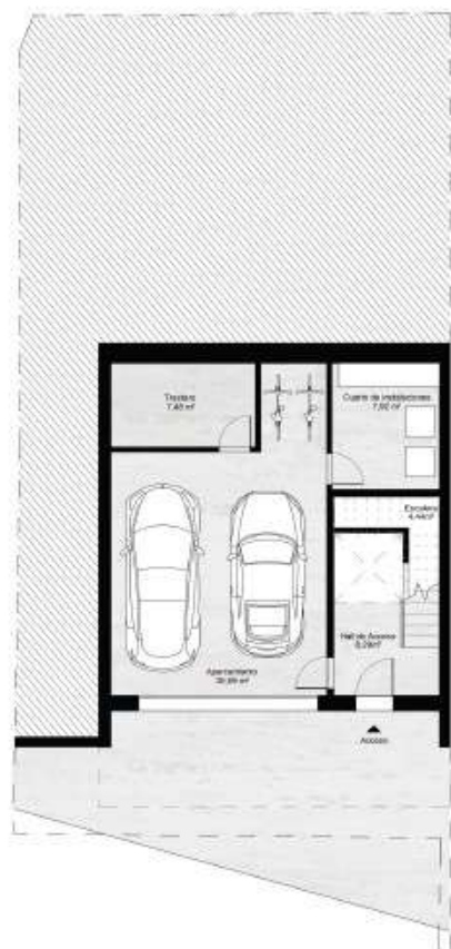
PLANTA SÓTANO
