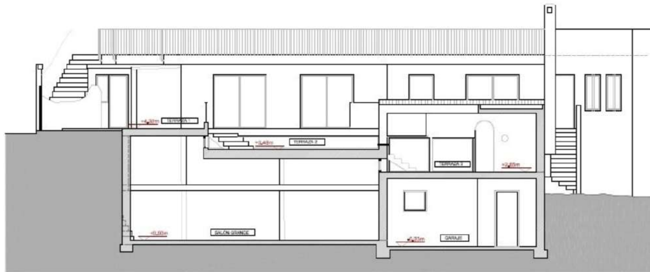
SECCIÓN C-C'
