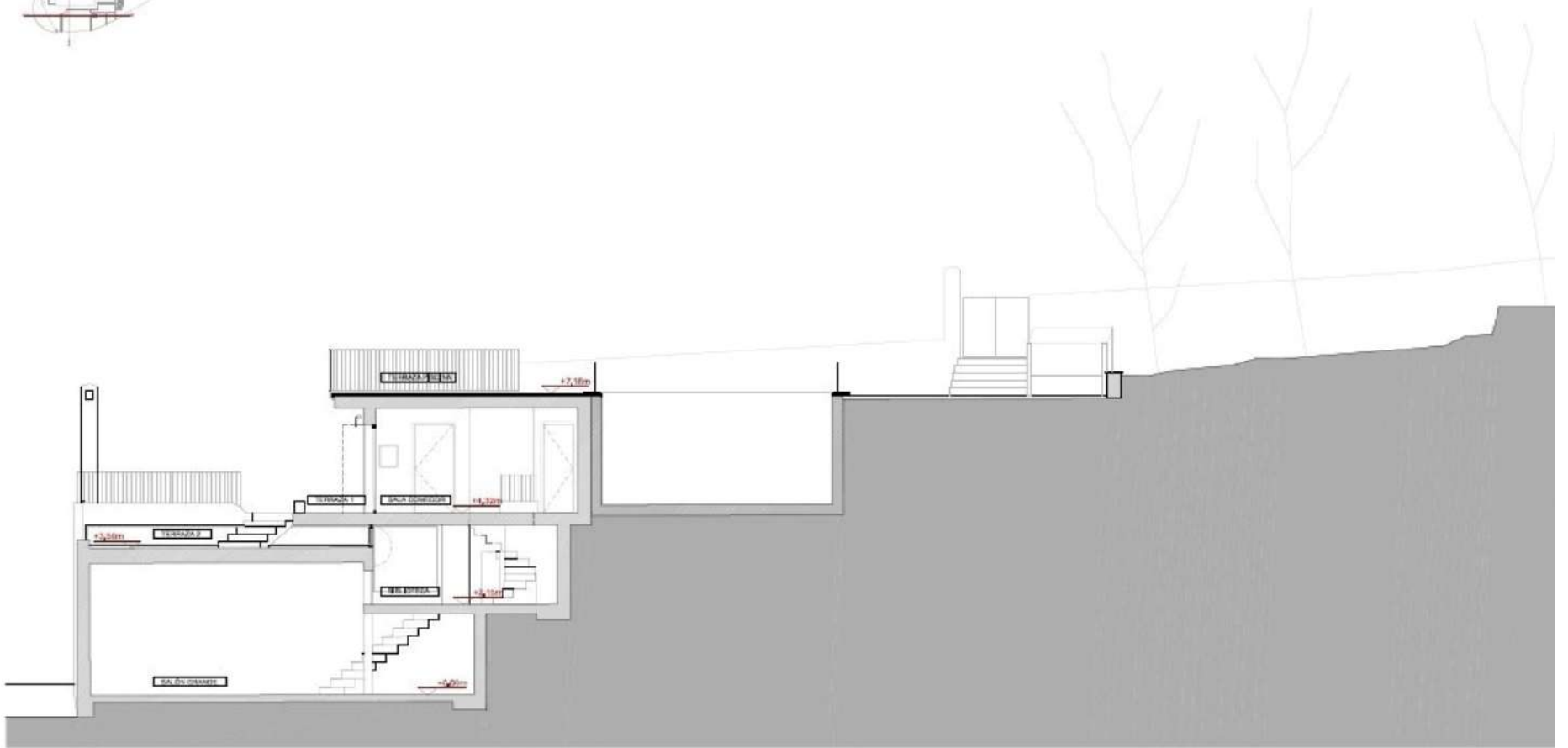
SECCIÓN A-A'
