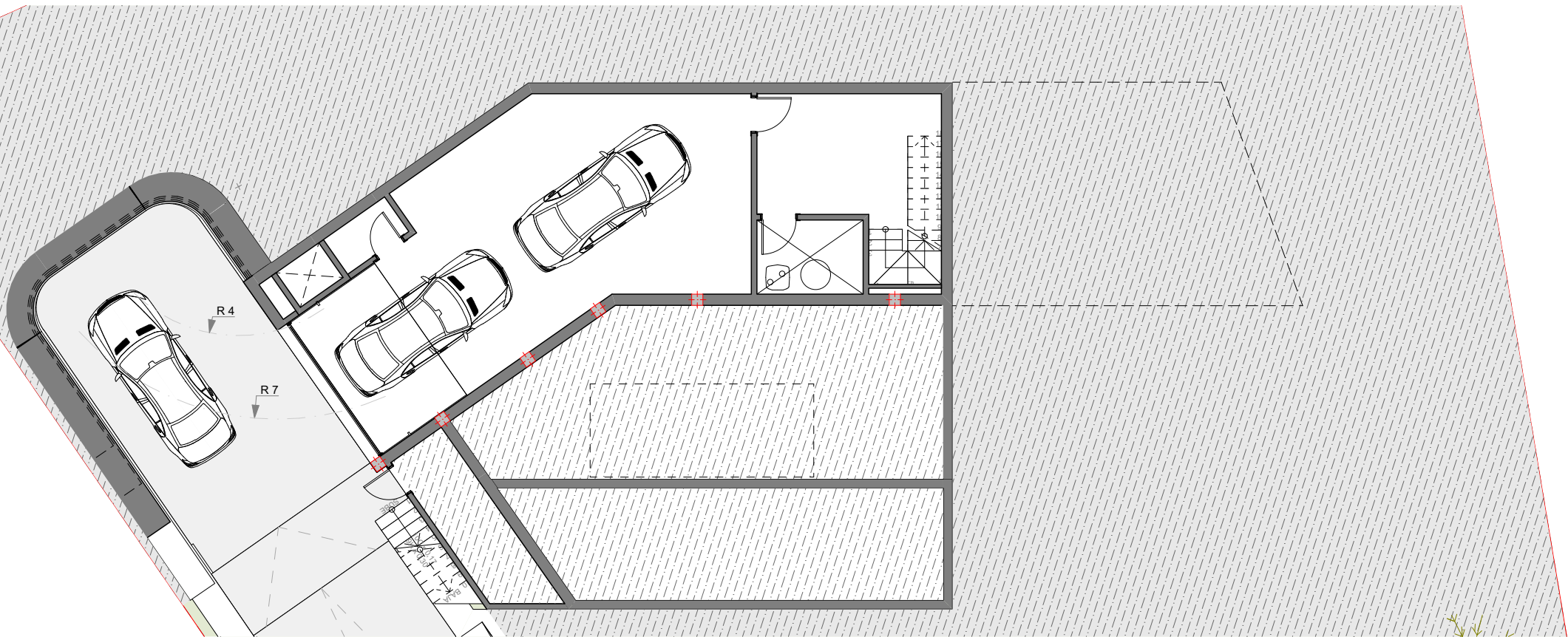
Planta Sotterrani
