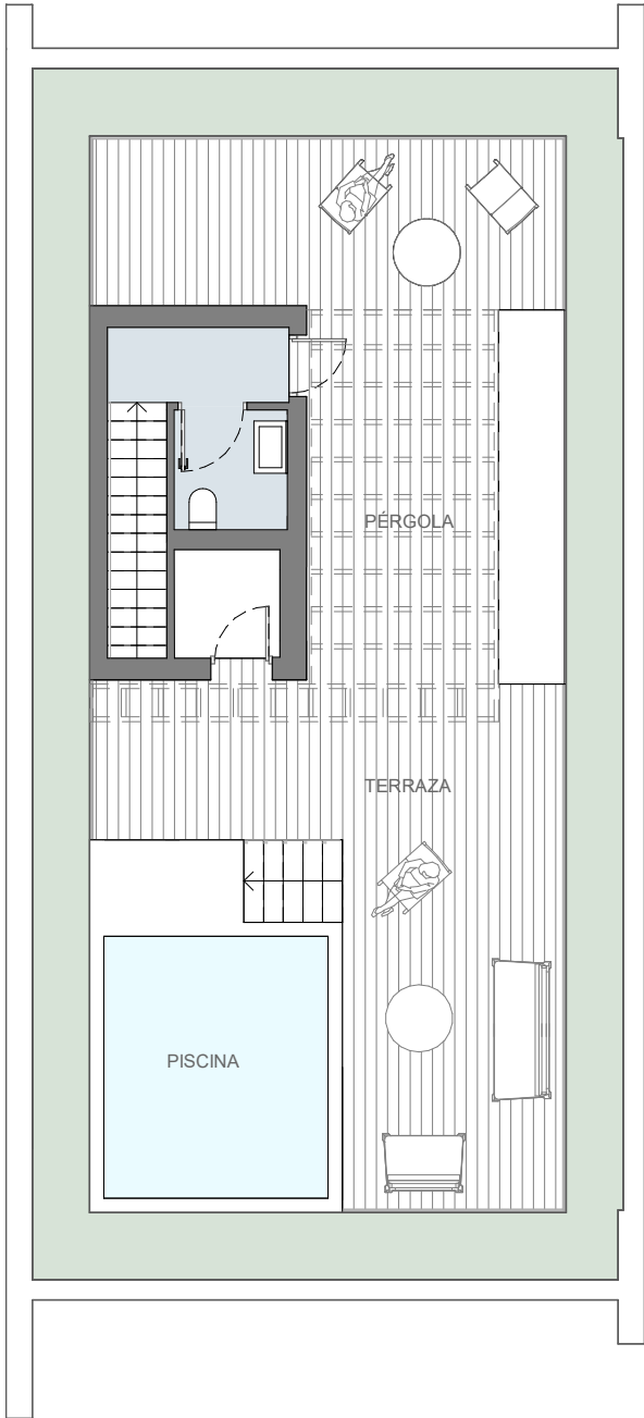
PLANTA CUBIERTA
