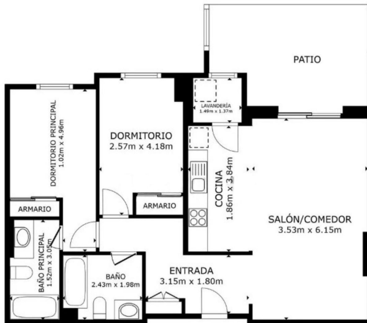
PLANTA
