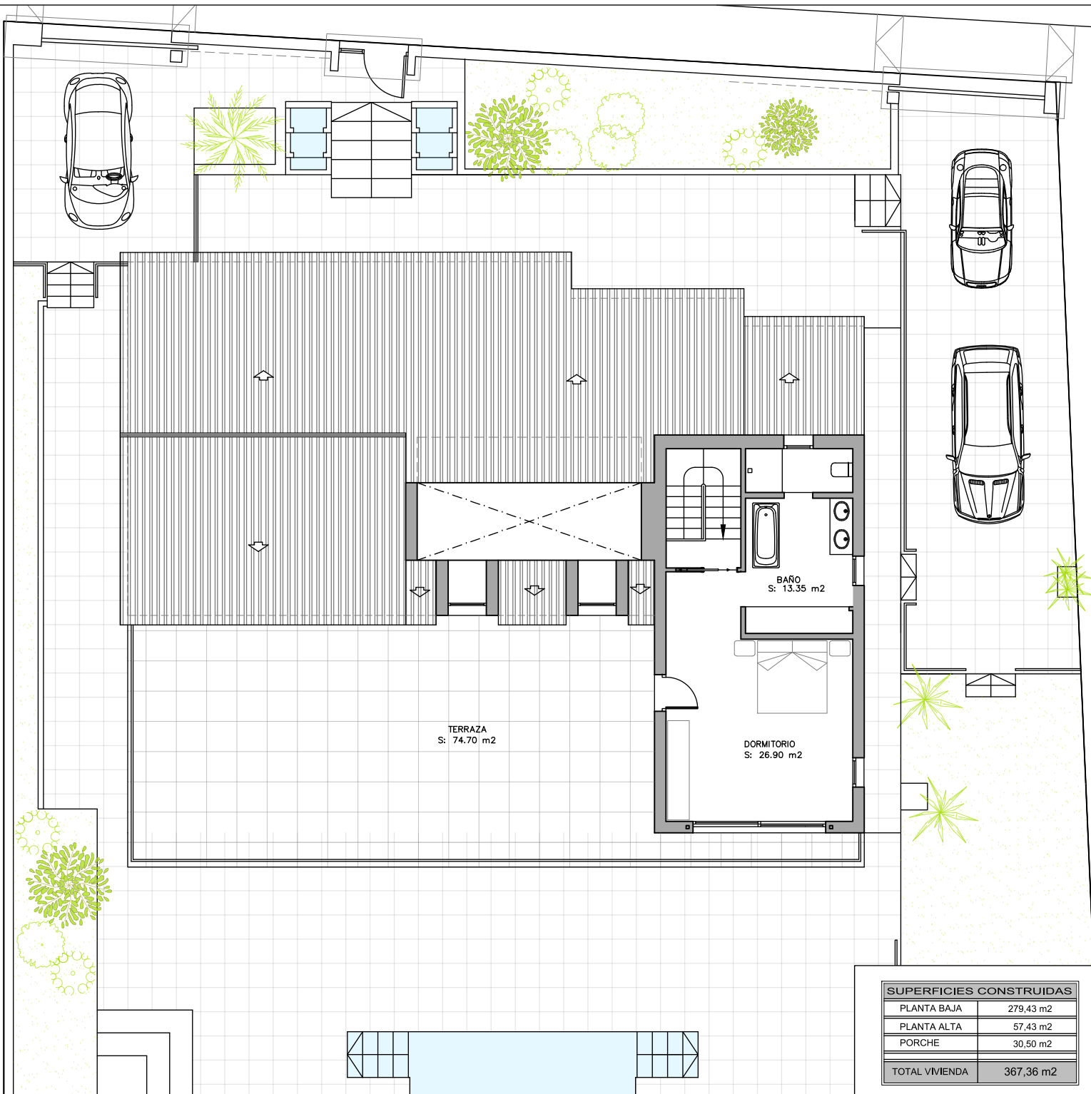
PLANO: PLANTA ALTA COTAS Y SUPERFICIES
