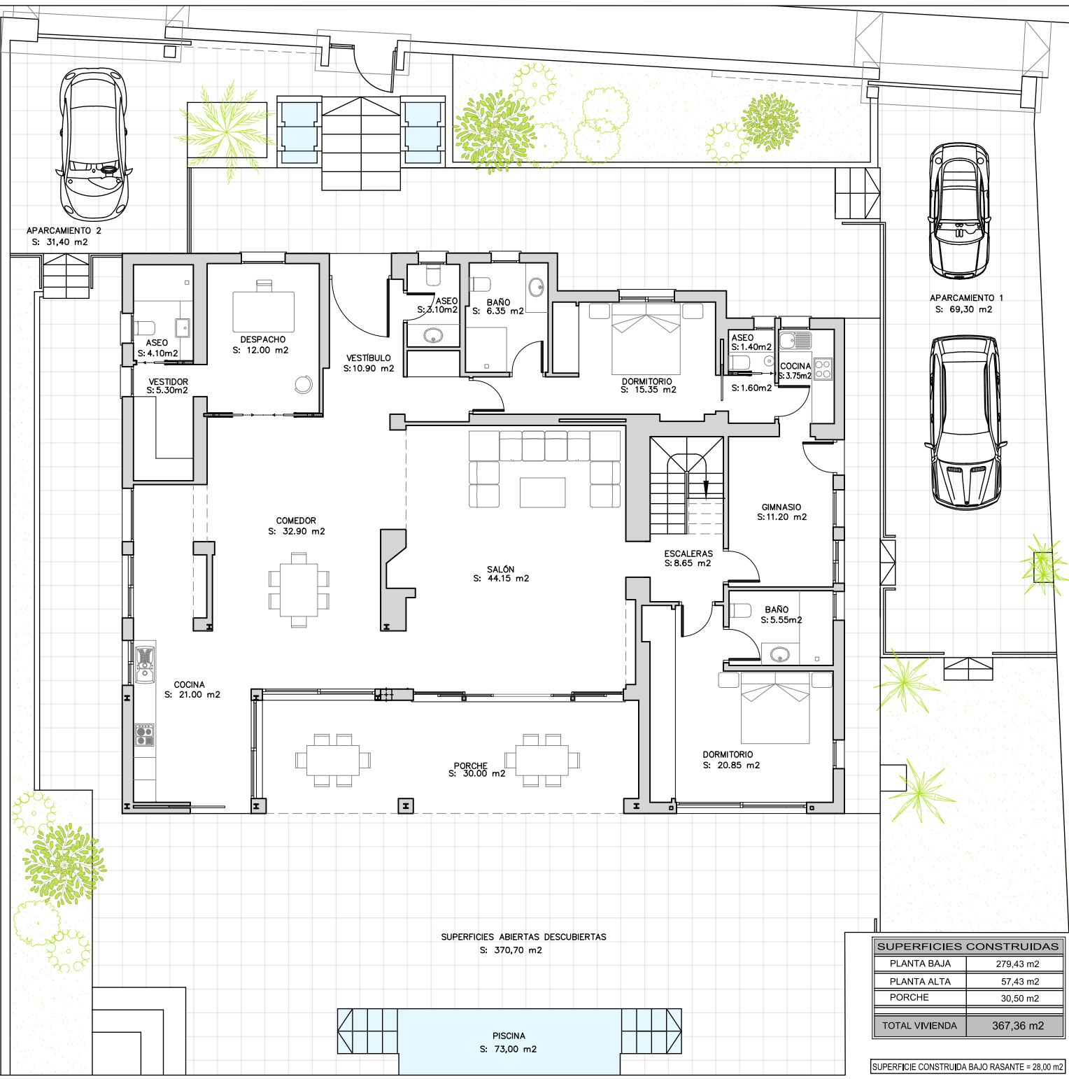
PLANO: PLANTA BAJA COTAS Y SUPERFICIES
