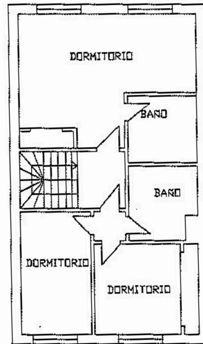
PLANTA PRIMERA
