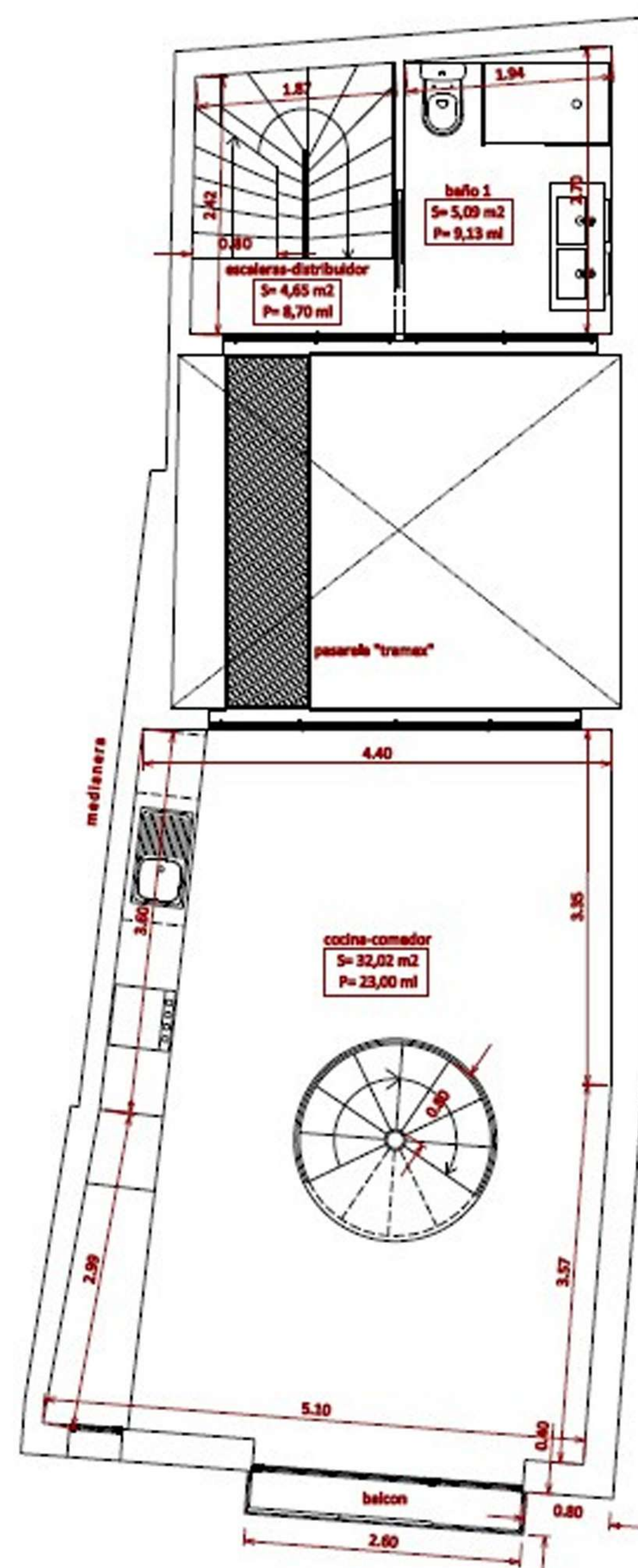
PLANTA PRIMERA
