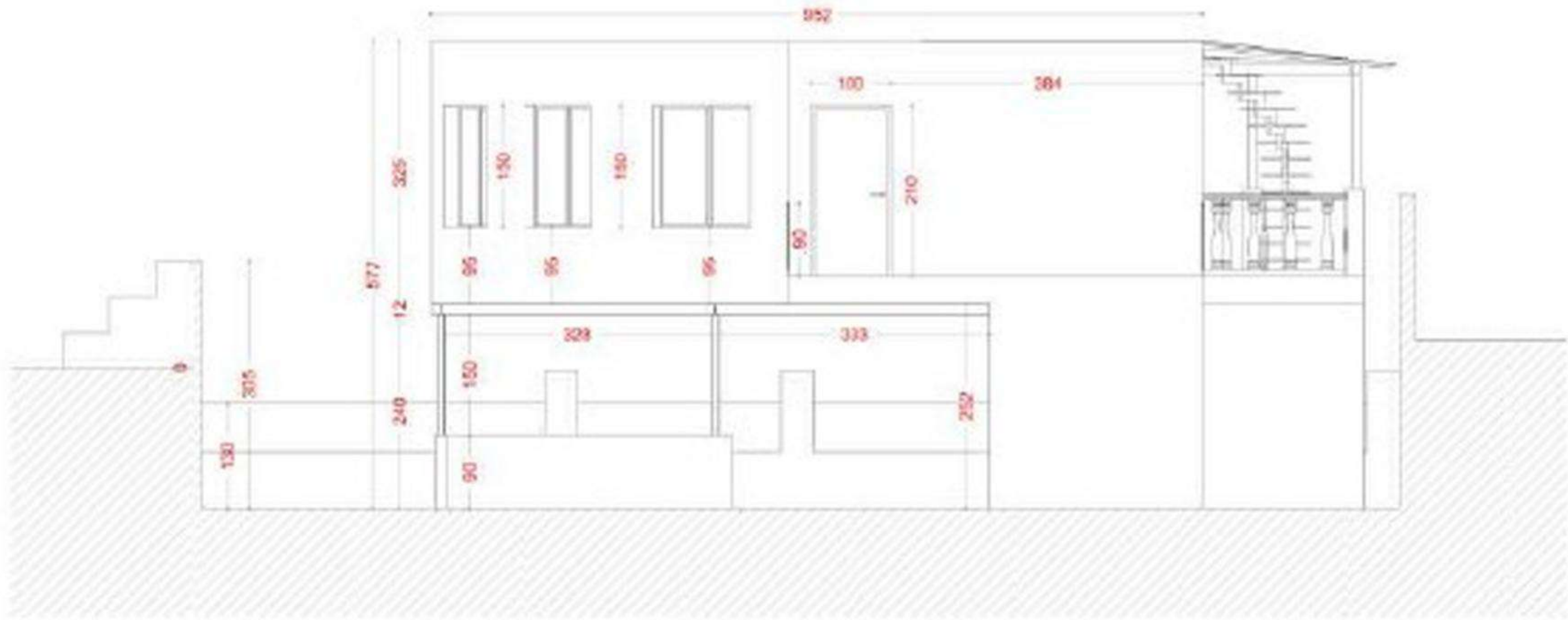
ALZADO SUR SOUTH ELEVATION
