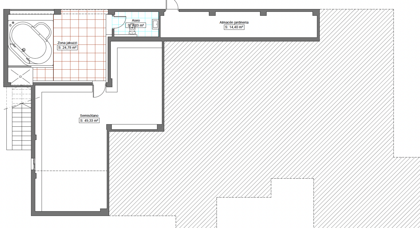
PLANTA SEMISOTANO
