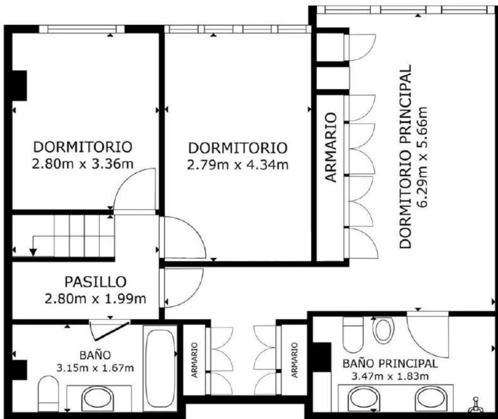
PLANTA 1
