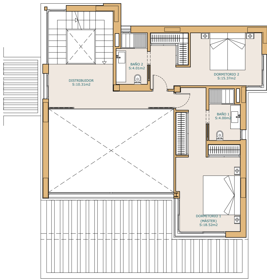
PLANTA PRIMERA
