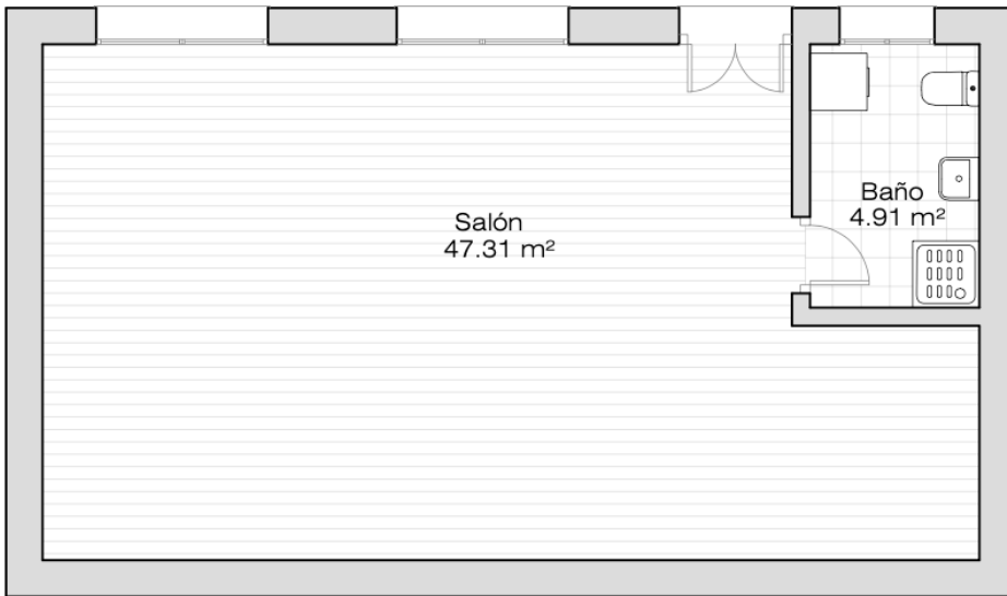
PLANTA SEMISÓTANO
