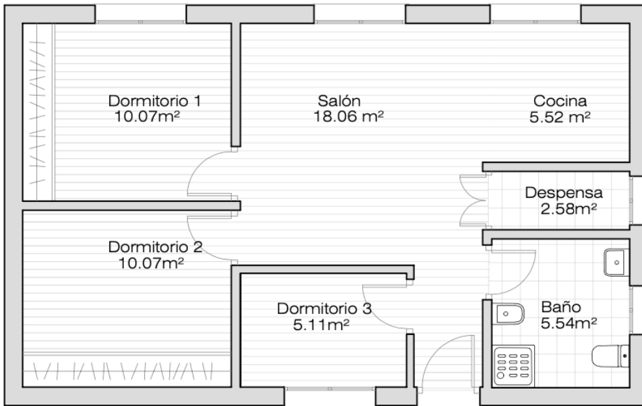
PLANTA BAJA
