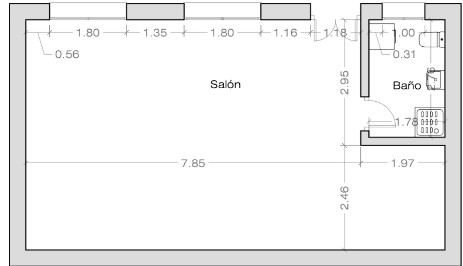
PLANTA SEMISÓTANO
