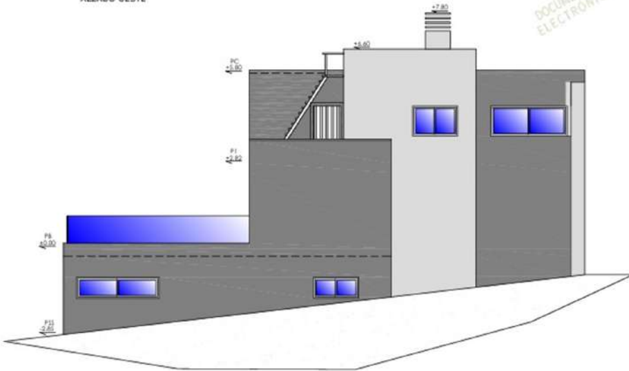
ALZADO OESTE
