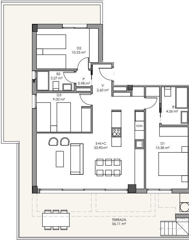
PLANTA CUBIERTA
