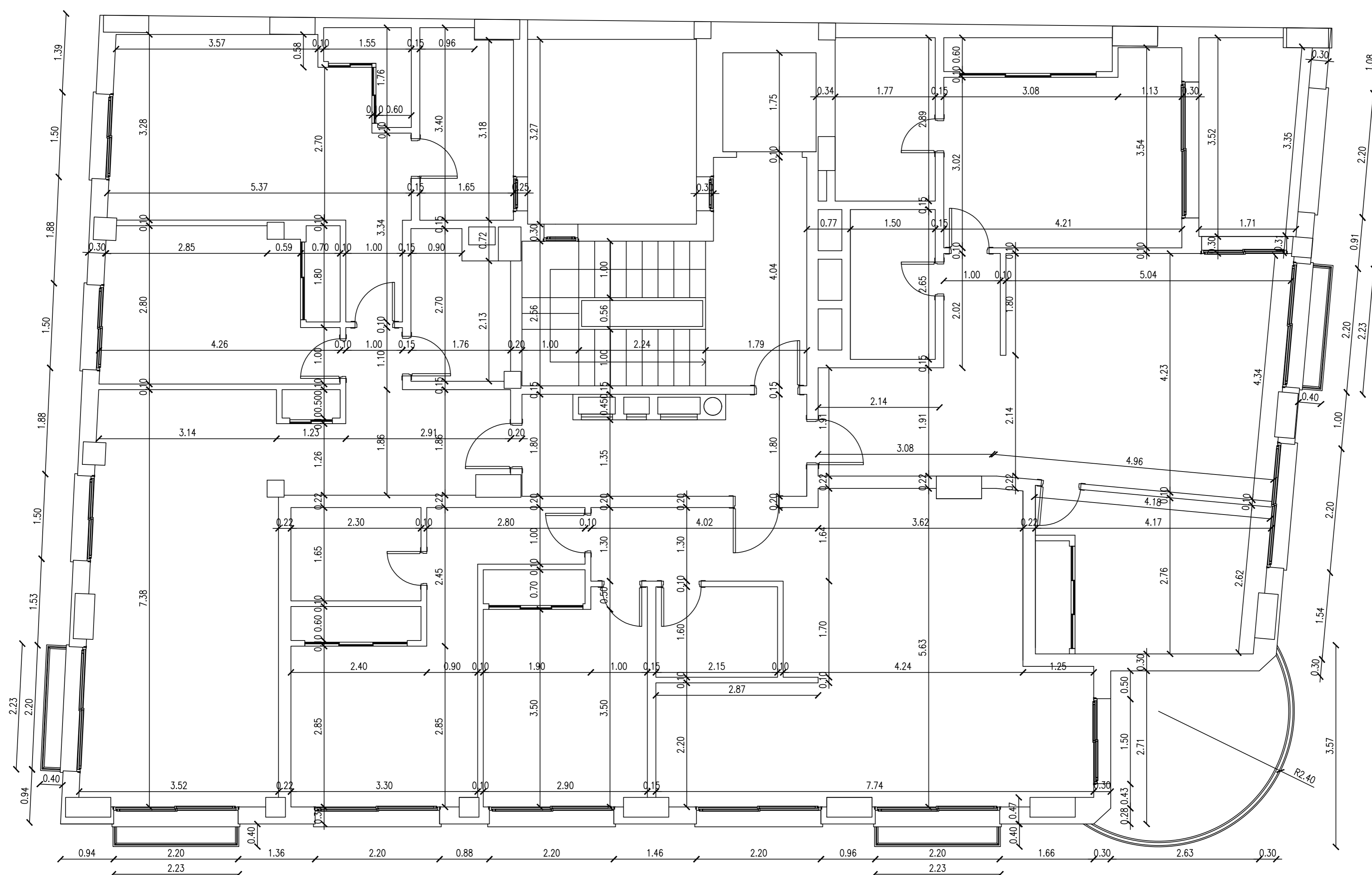
PLANTAS PRIMERA ACOTADO
