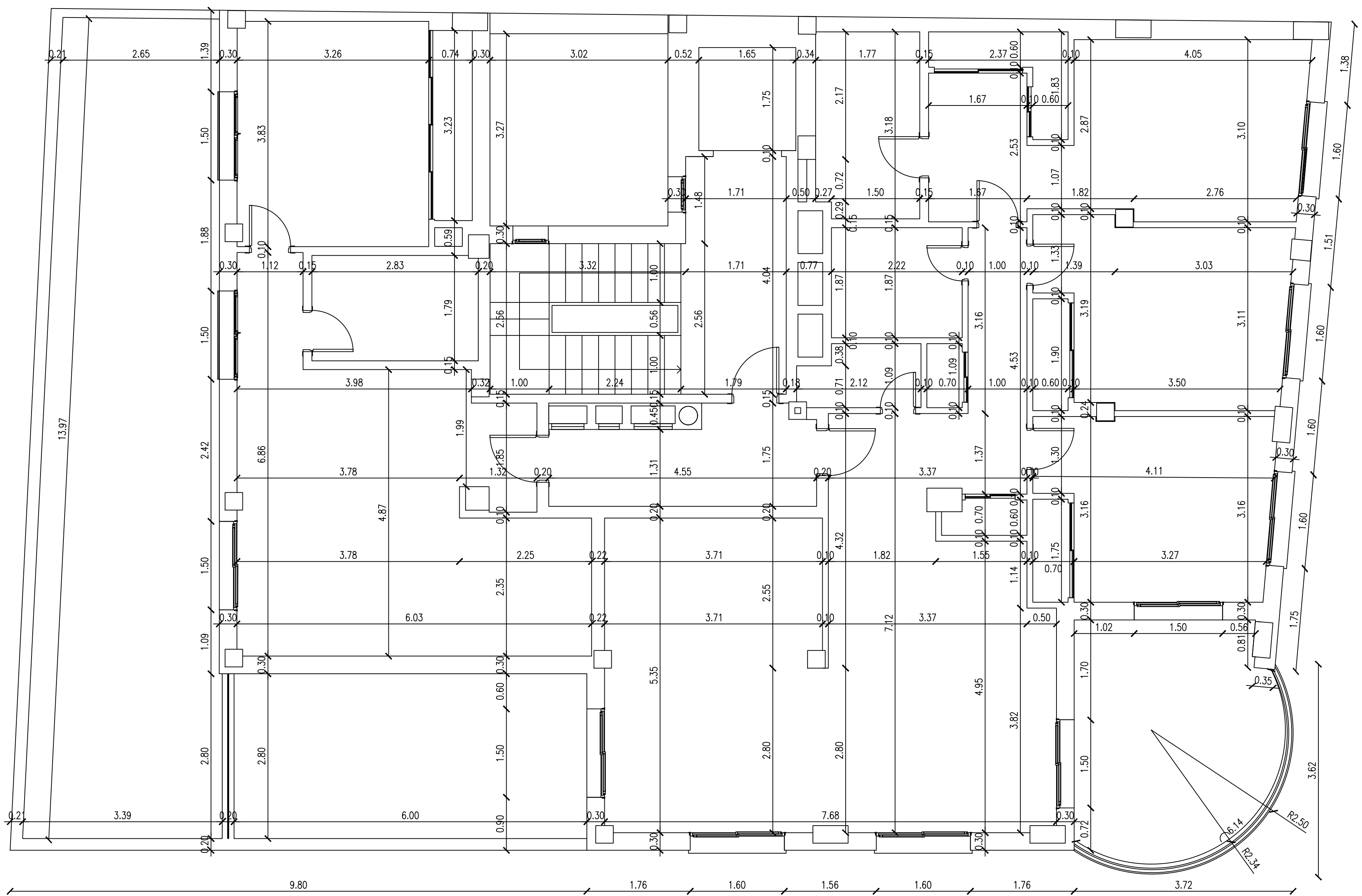
PLANTA CUARTA ACOTADO
