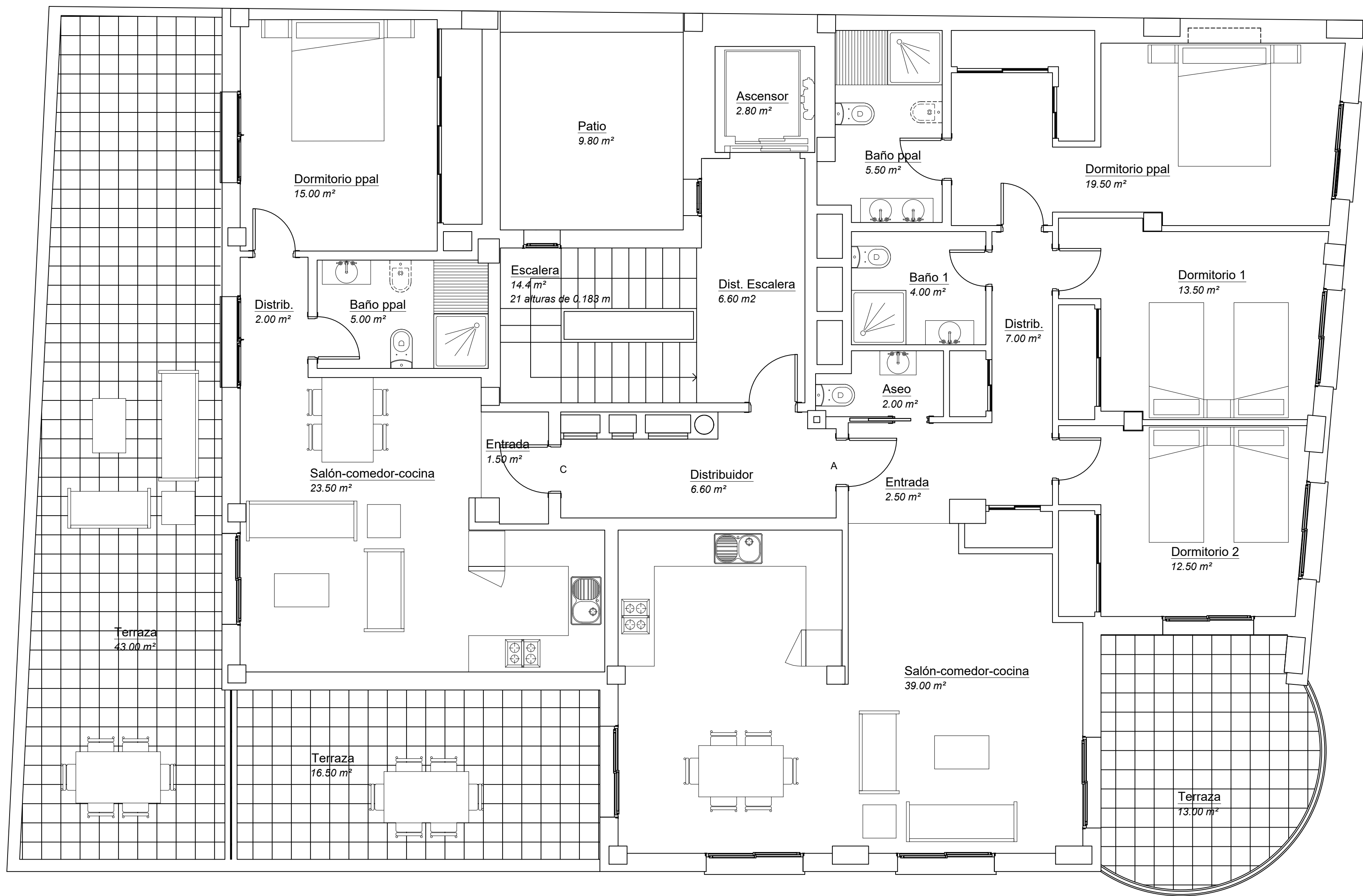
PLANTA CUARTA DISTRIBUCIÓN
