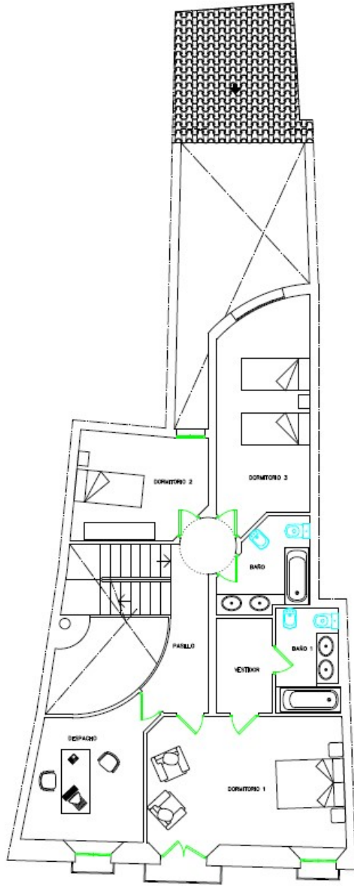
PLANTA ALTA
