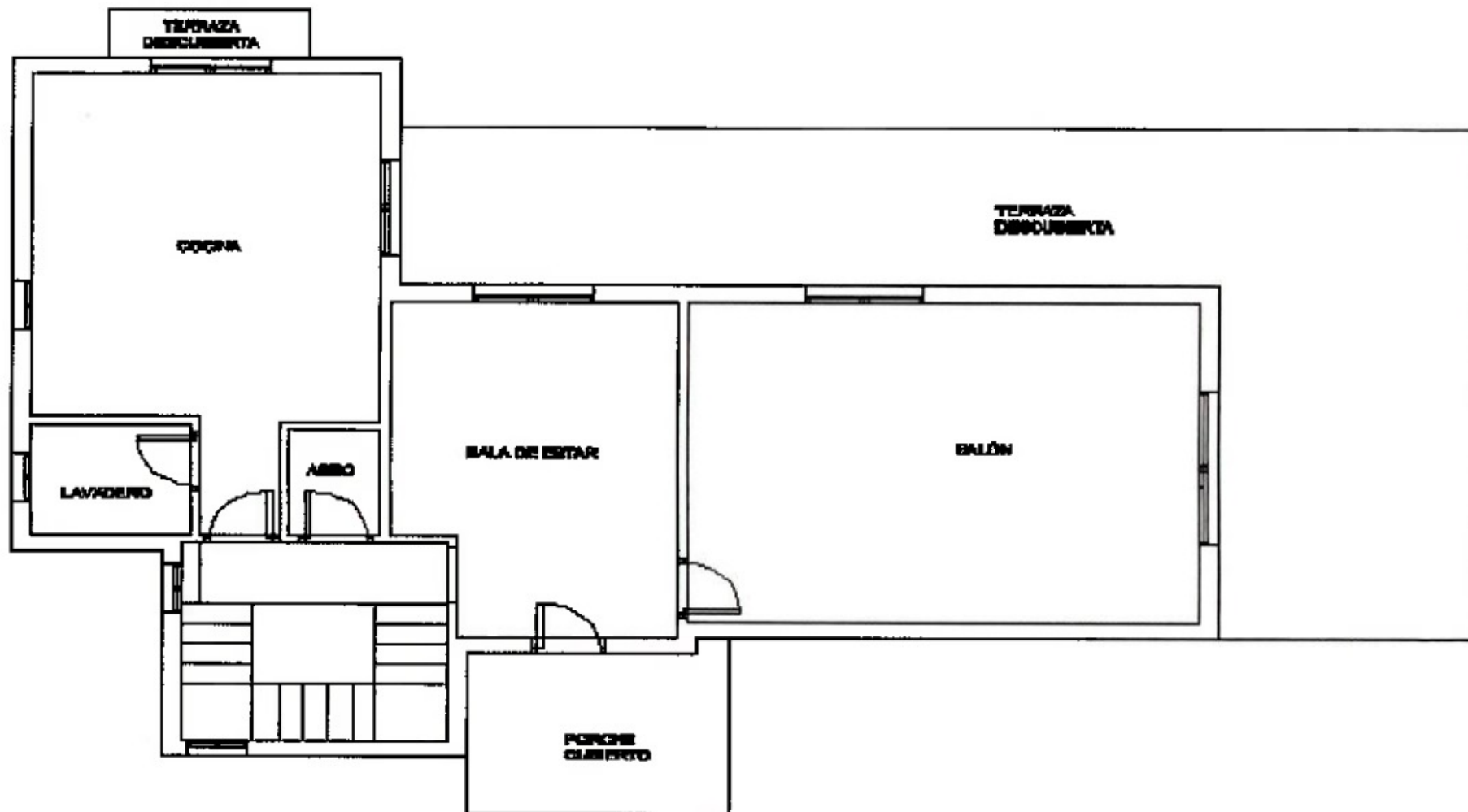
PLANTA ALTA
