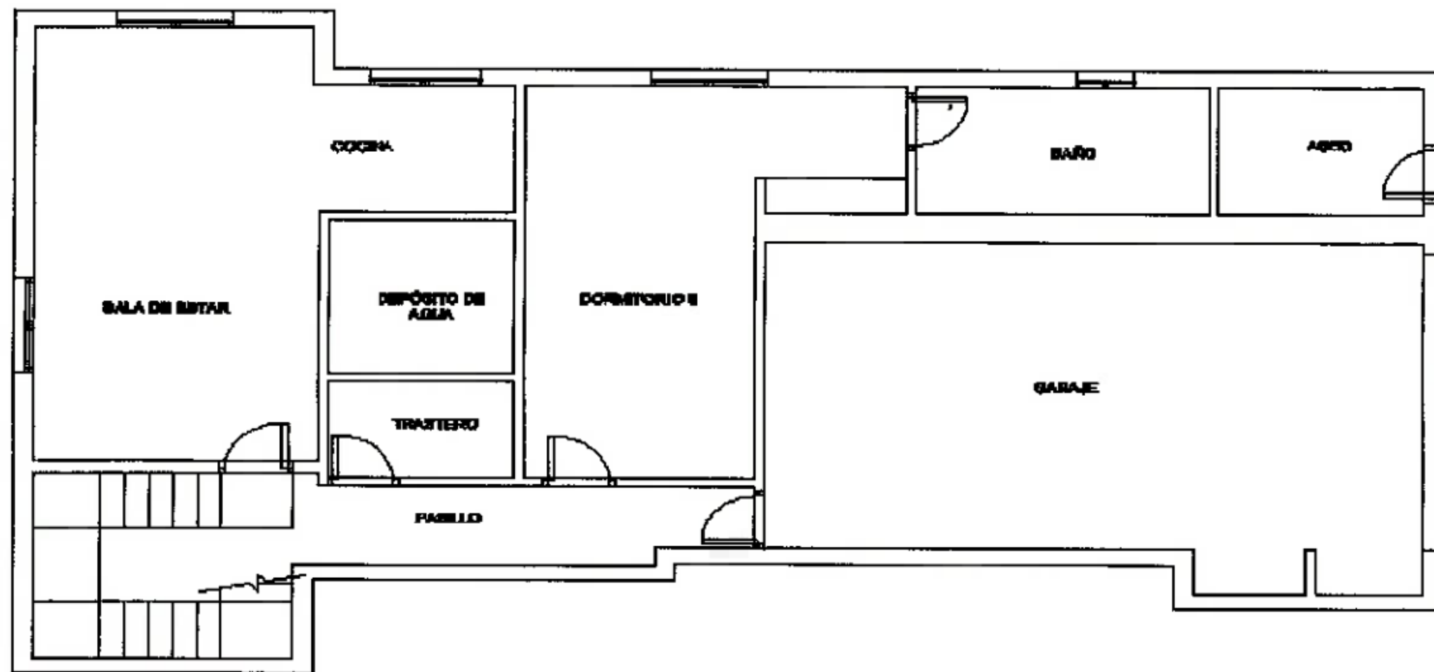
PLANTA BOTANO
