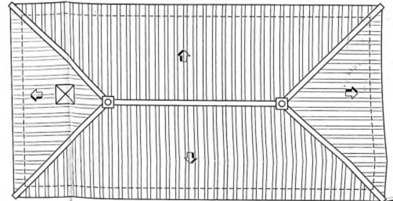
CUBIERTA GARAJE Pte. 35%
