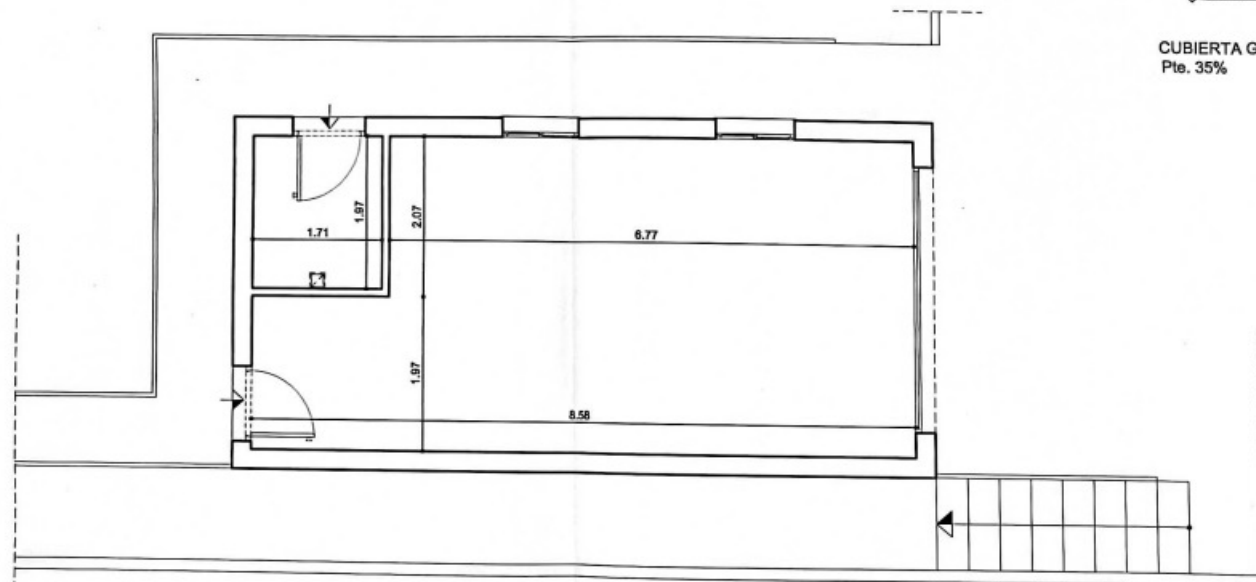
PLANTA DE GARAJE
