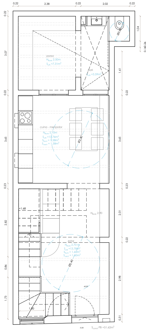
PLANTA BAIXA
