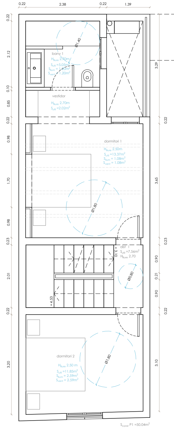
PLANTA PRIMERA
