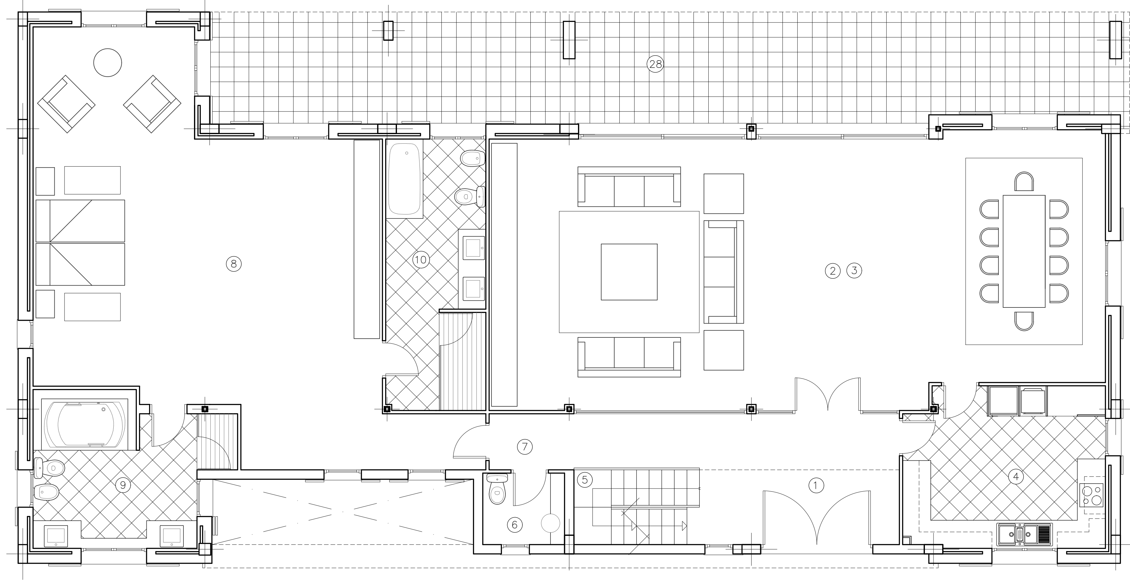
DISTRIBUCION PLANTA BAJA SUPERFICIE CONSTRUIDA 50% TC 243.73 m2
