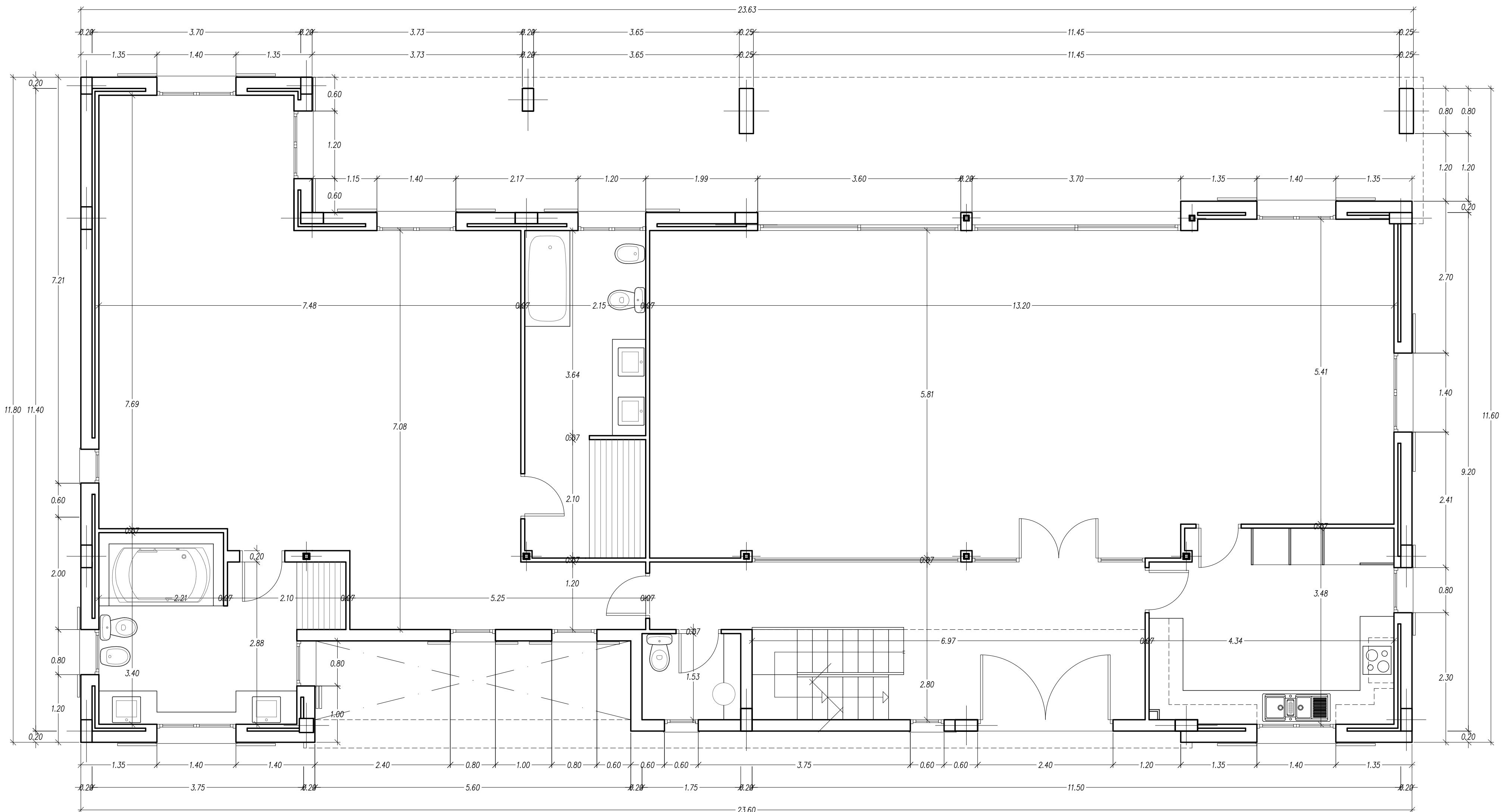
COTAS PLANTA BAJA
