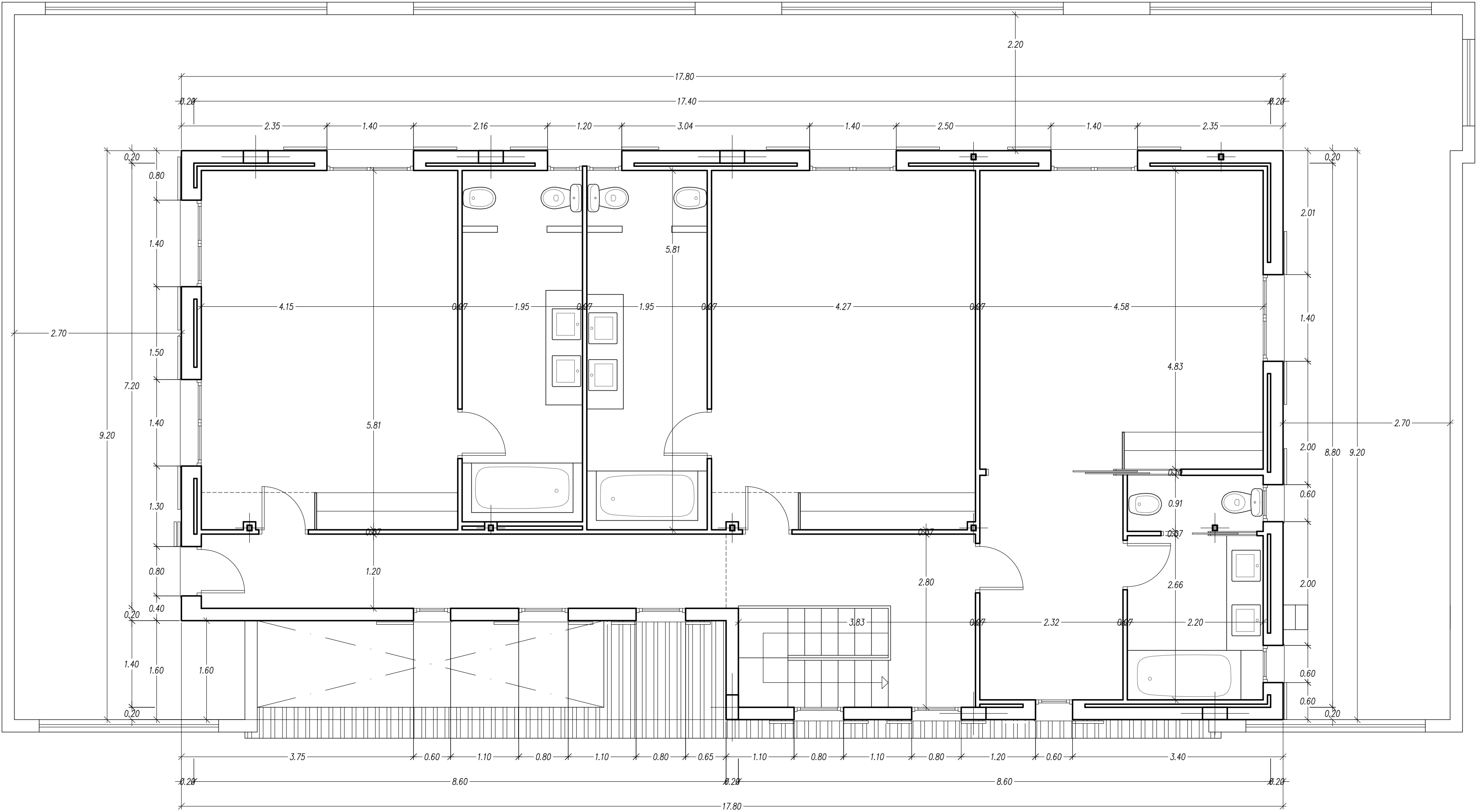
COTAS PLANTA PISO
