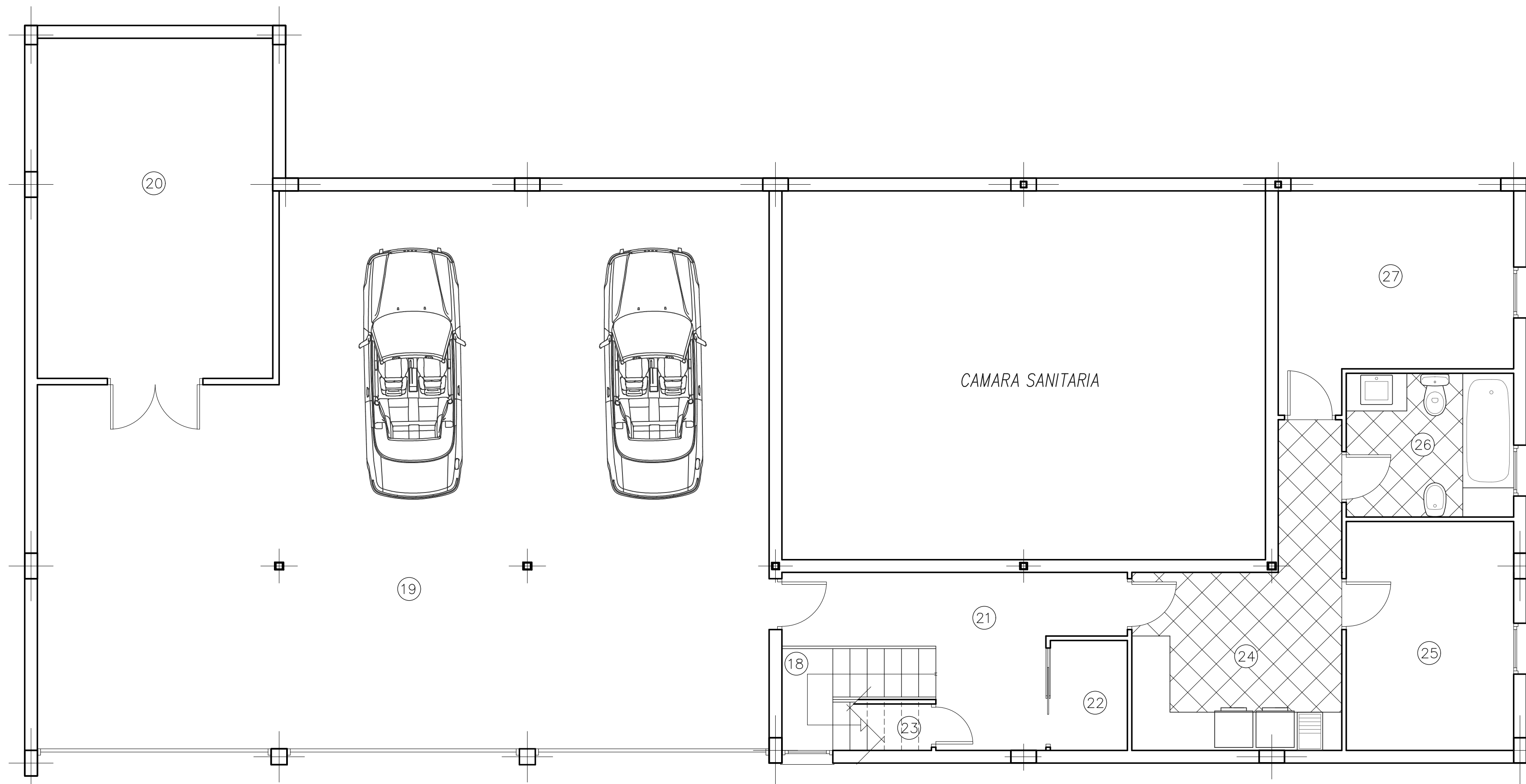
DISTRIBUCION PLANTA SOTANO SUPERFICIE CONSTRUIDA 50% TC 182.92 m2
