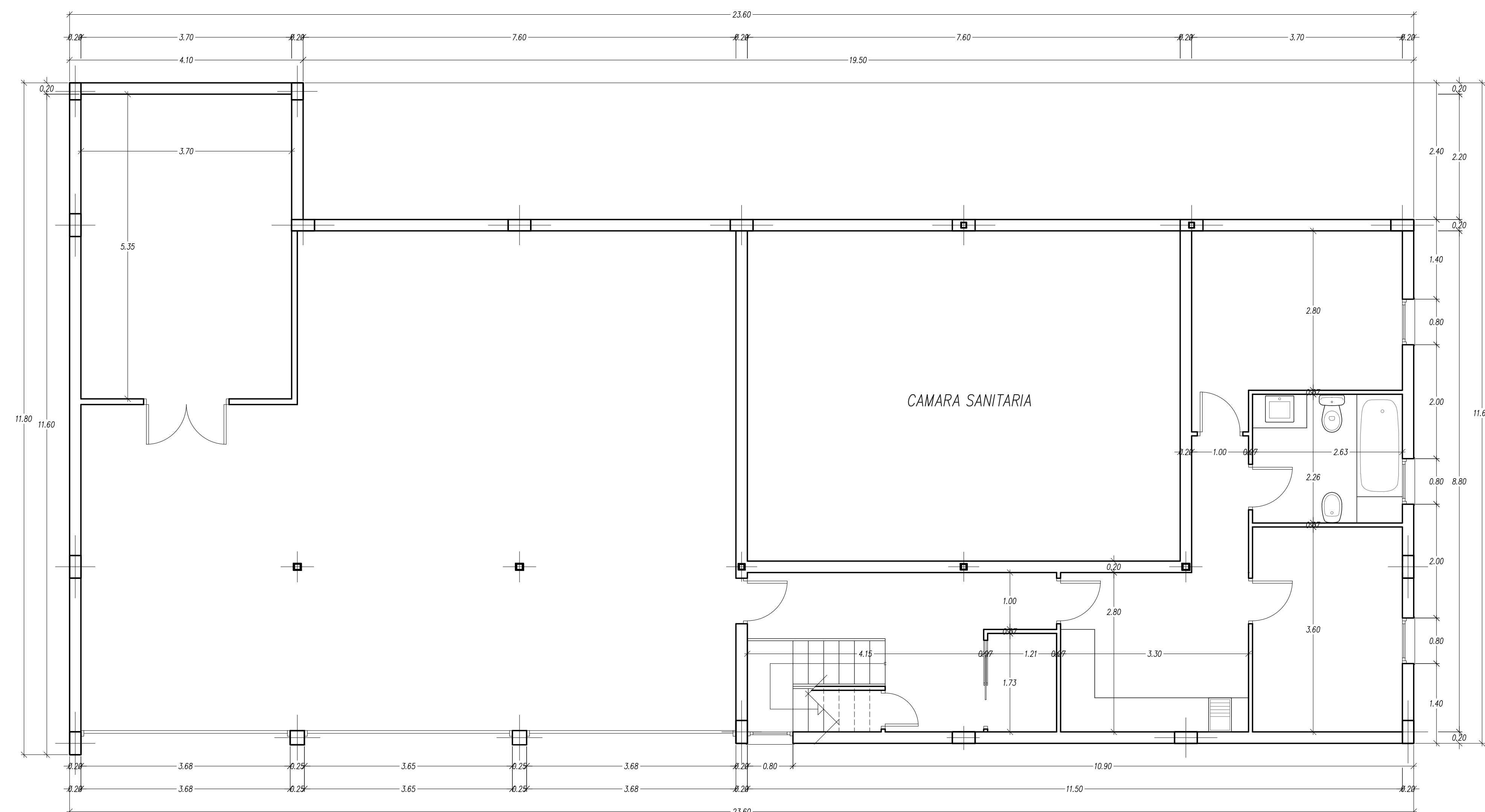
COTAS PLANTA SOTANO
