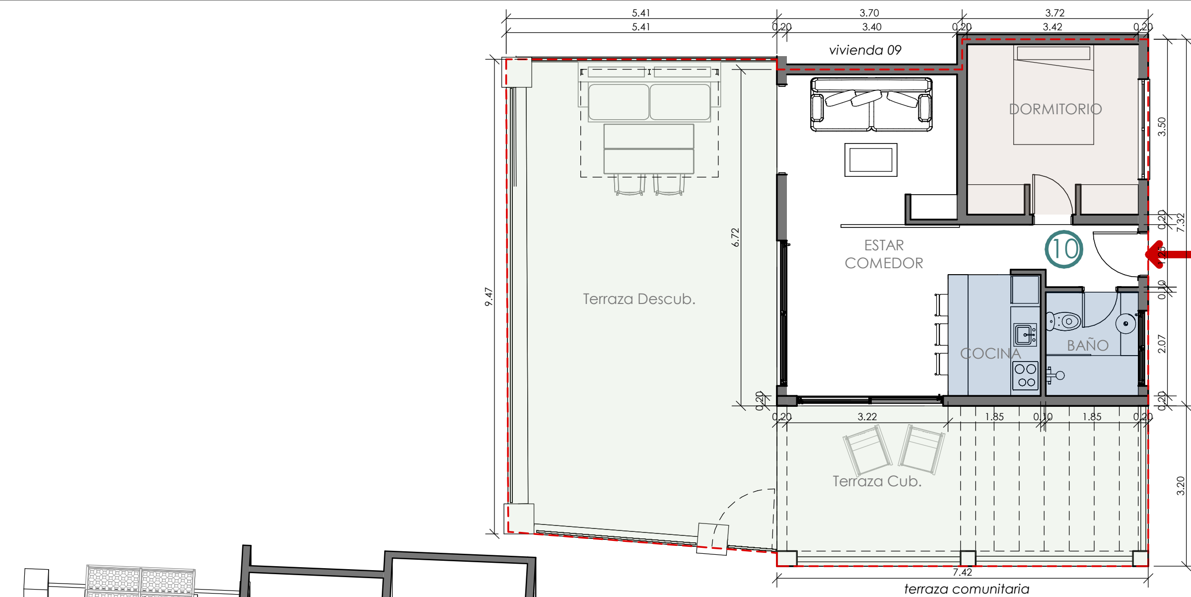
PLANTA
