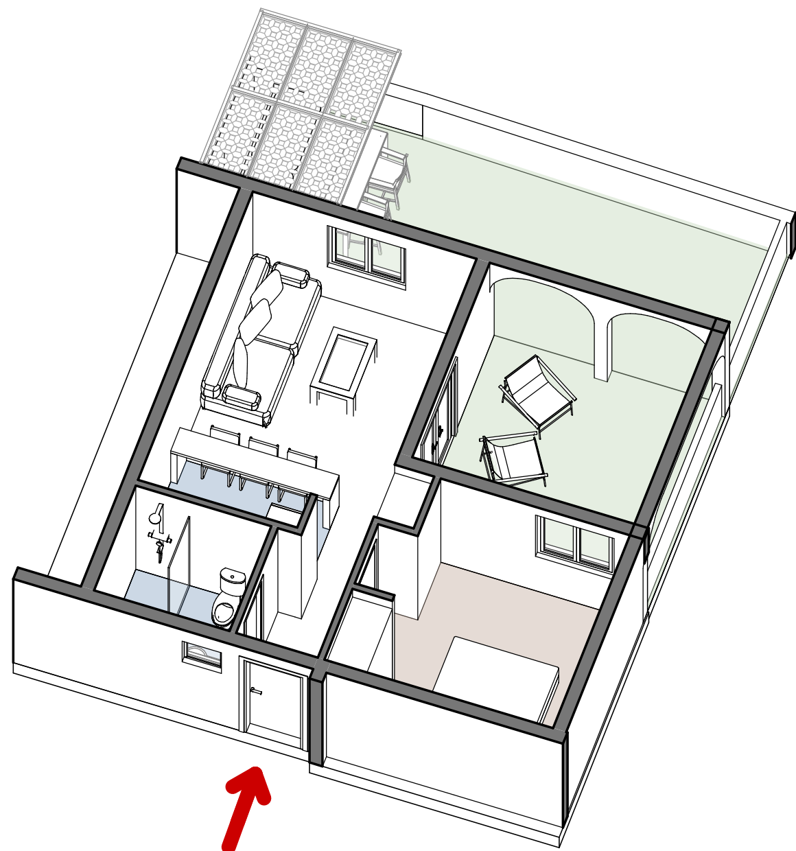
AXONOMETRÍA
