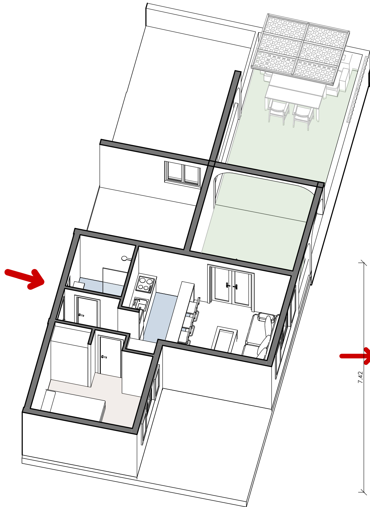
AXONOMETRÍA
