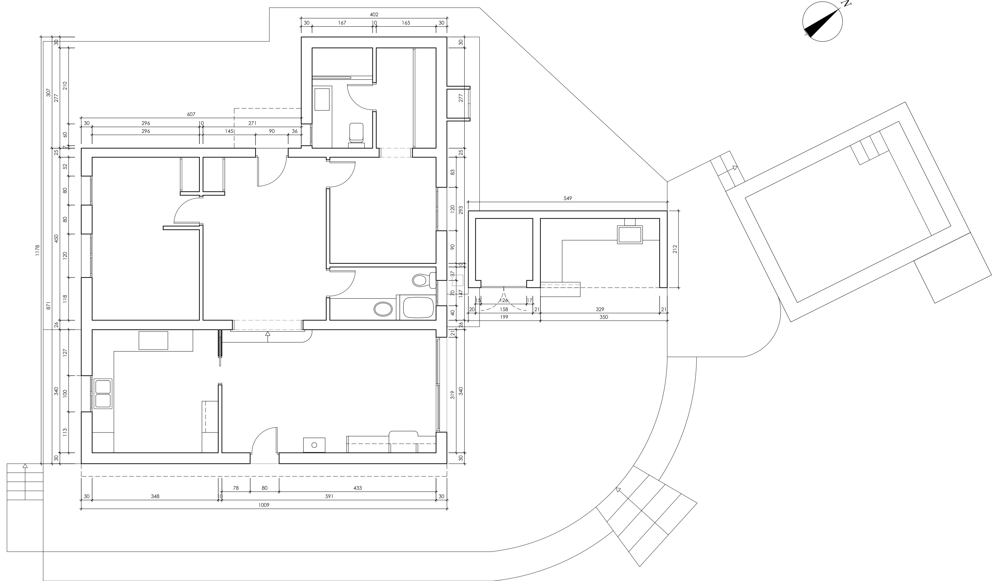
PLANTA COTAS VIVIENDA
