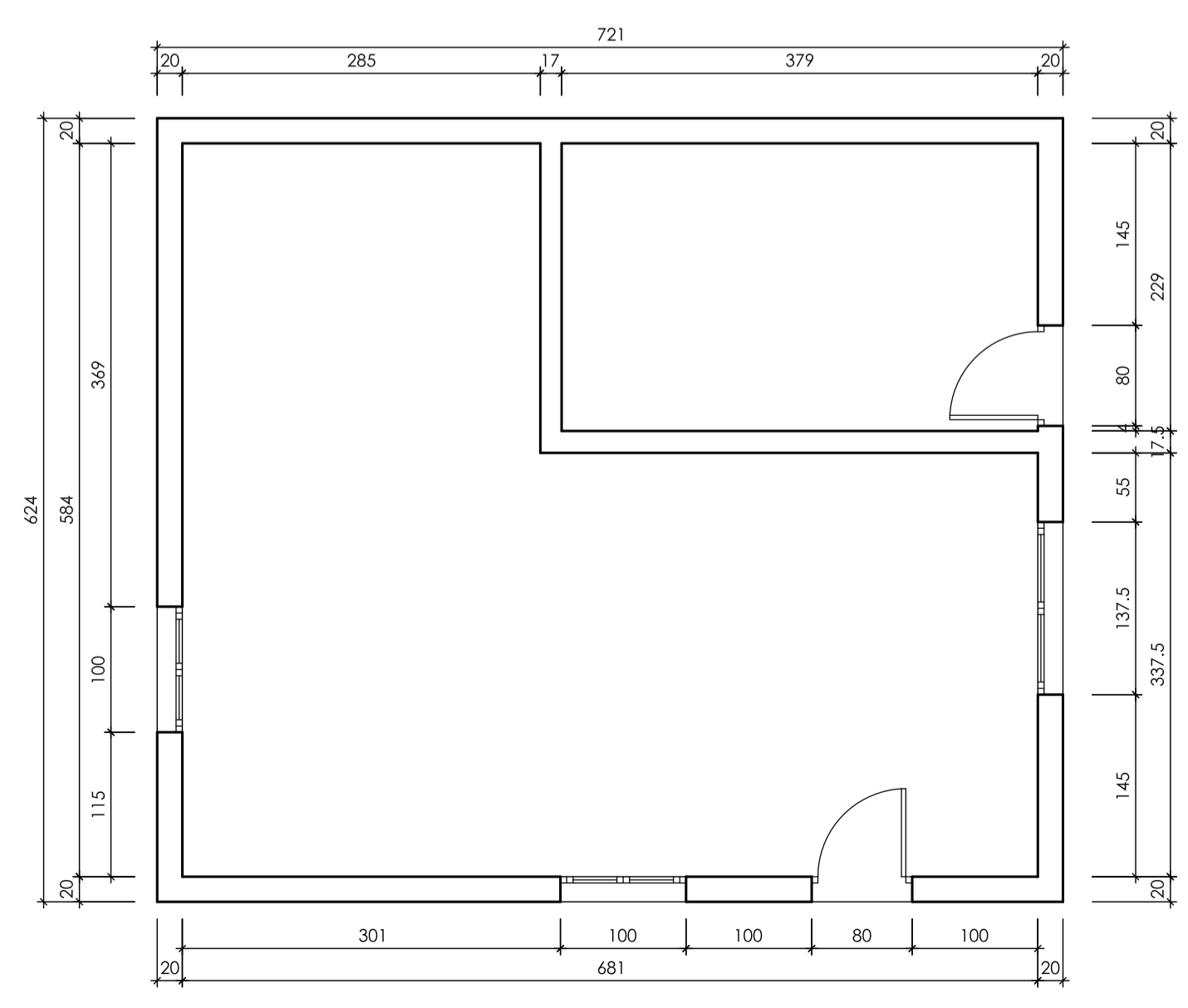
PLANTA COTAS ALMACEN
