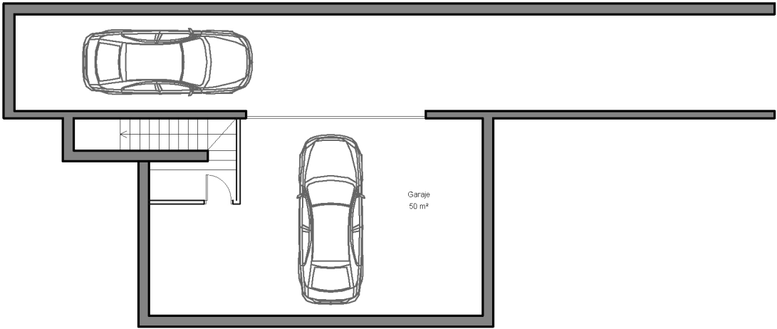
PLANTA SOTANO
