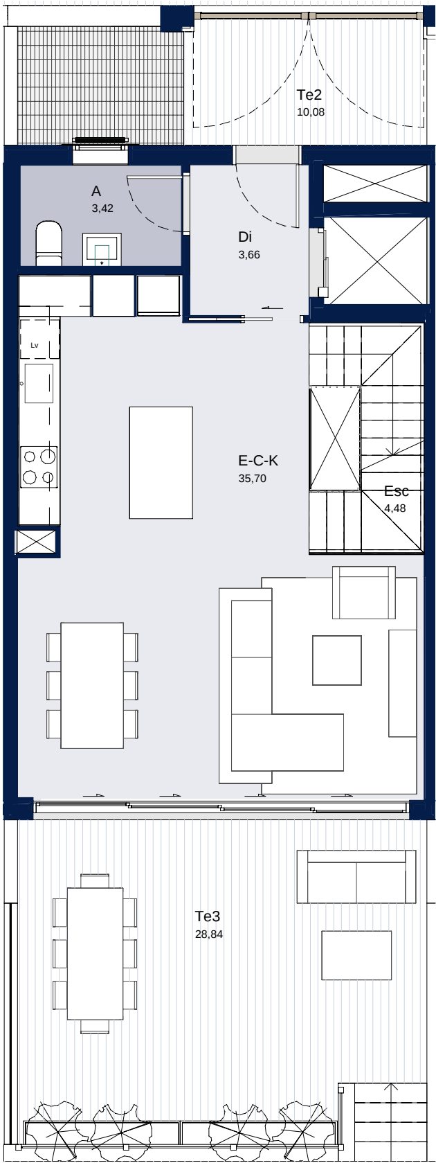
Planta Baja
