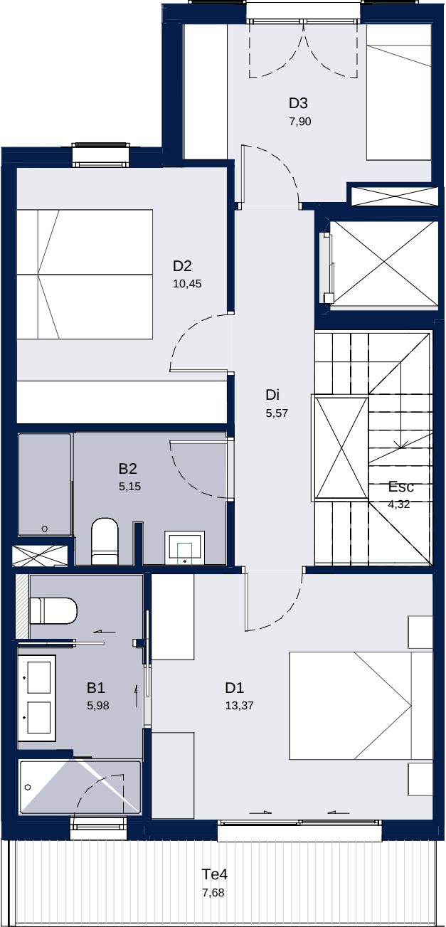
Planta Primera
