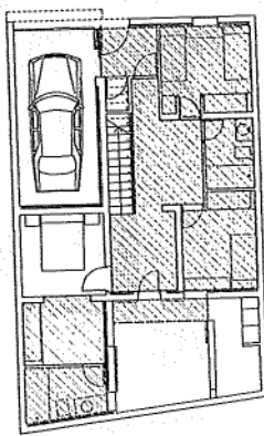
PLANTA BAIXA FALS SOSTRE
