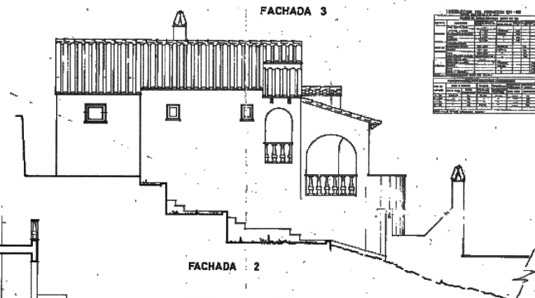
FACHADA 3
