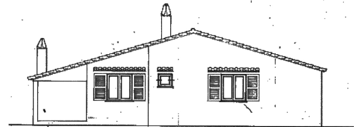
FACHADA 3
