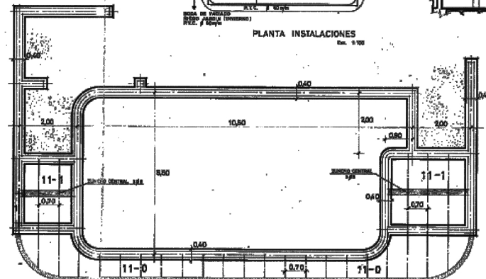
P. CIMENTACION PISCINA
