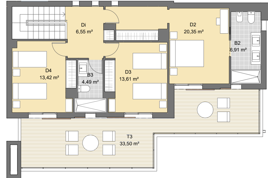
PLANTA PRIMERA
