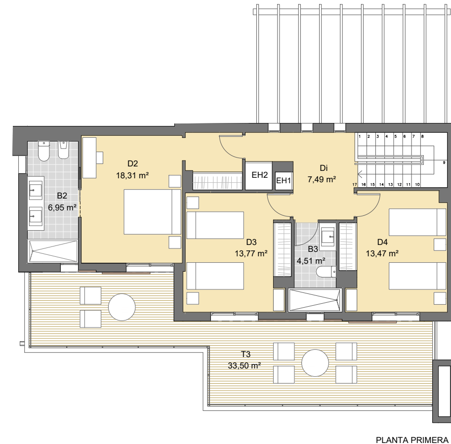
PLANTA PRIMERA
