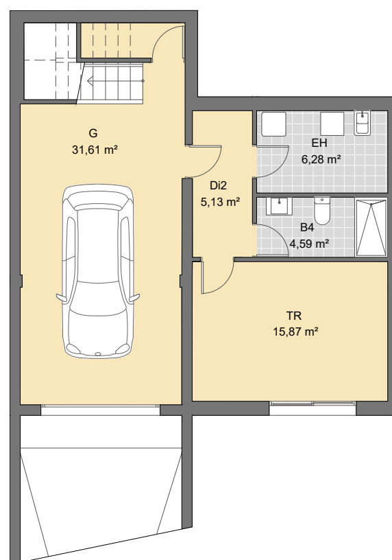
PLANTA SÓTANO
