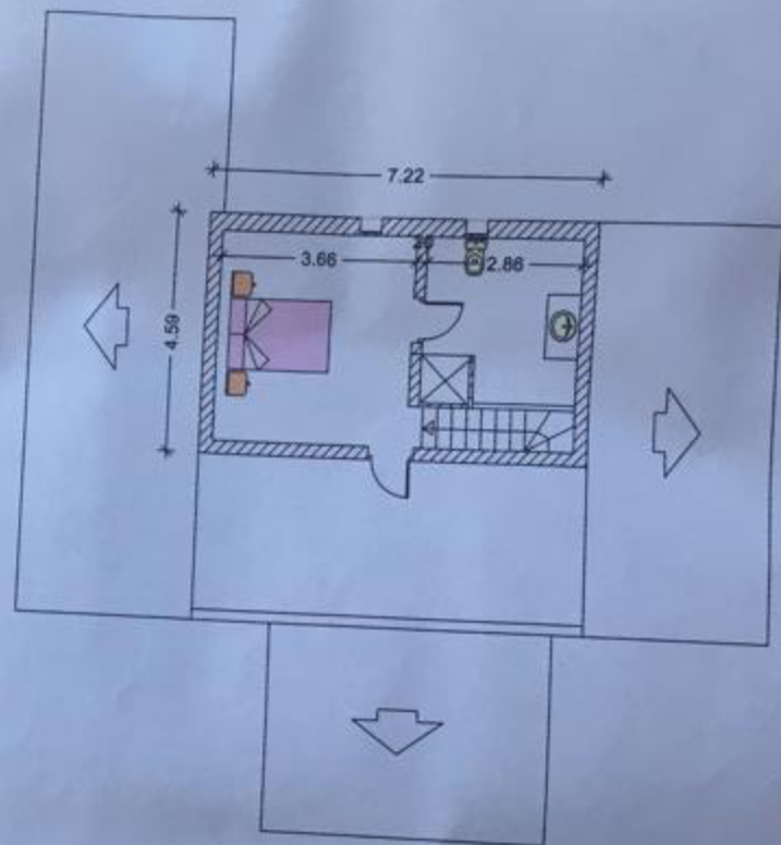
PLANTA PISO VIVIENDA
